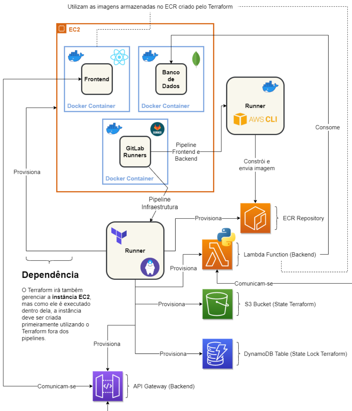
Figura 2 - Diagrama de Deploy - Veículos via Montadora
