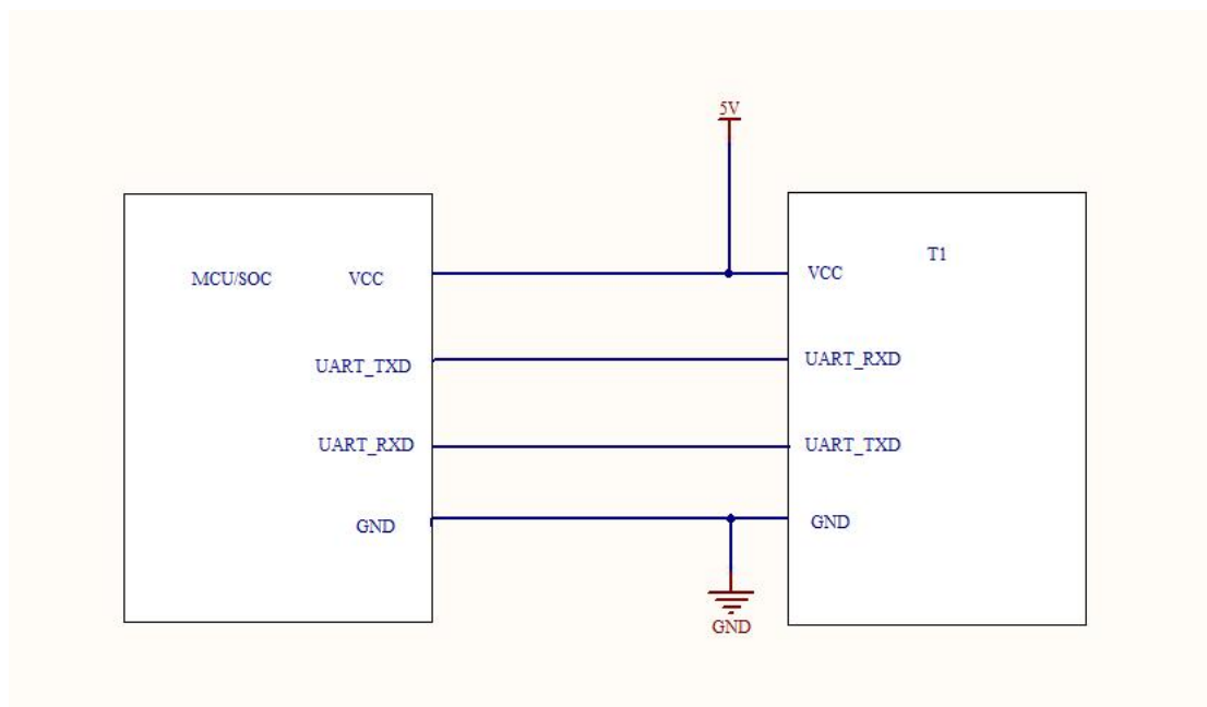
图3 UART 通讯模式电路图
