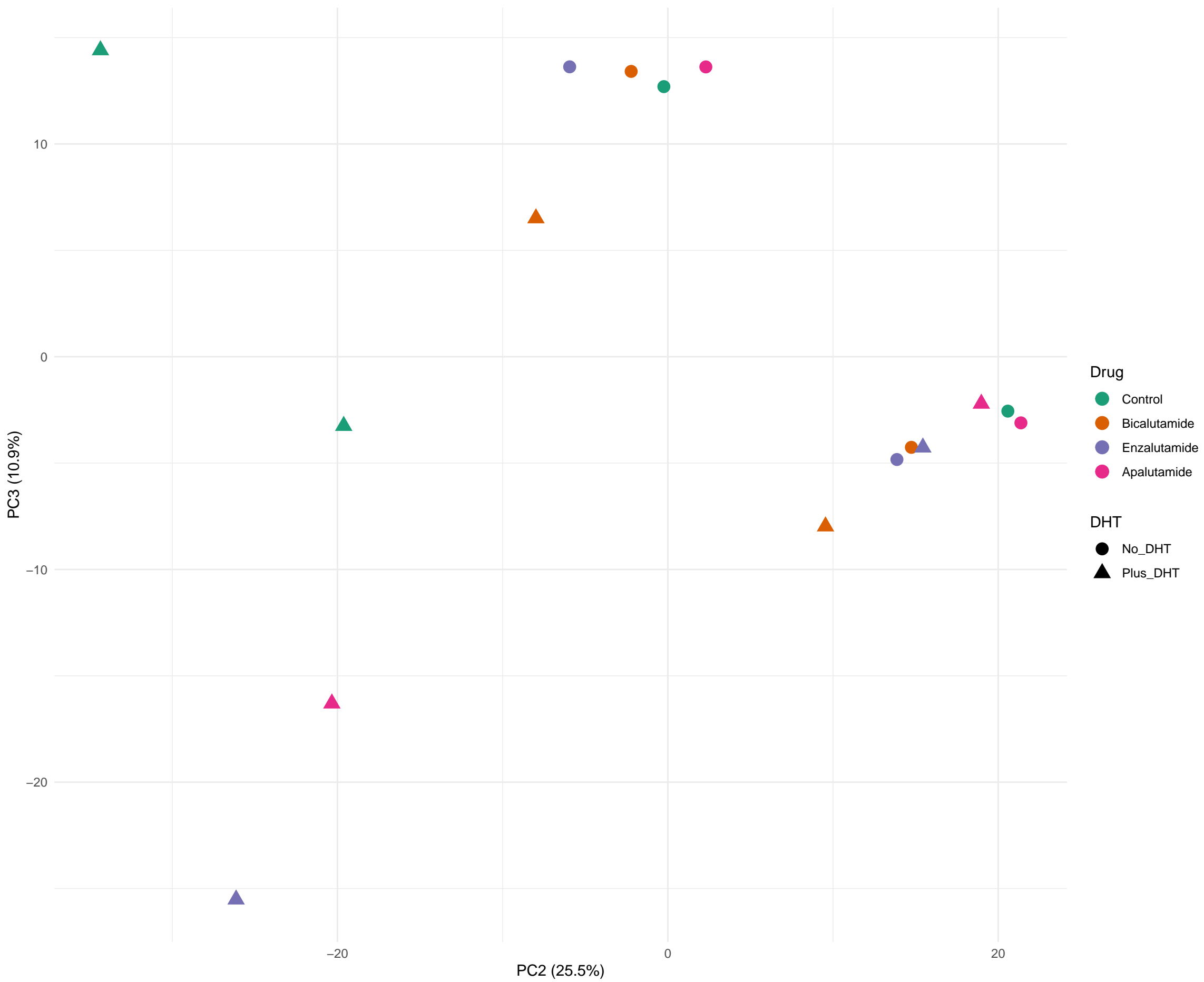
PCA: PC2 vs PC3
