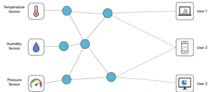
Figura 2.1: Una rete con dei Publisher (sensori), dei Broker e dei Subscriber (utenti finali)
