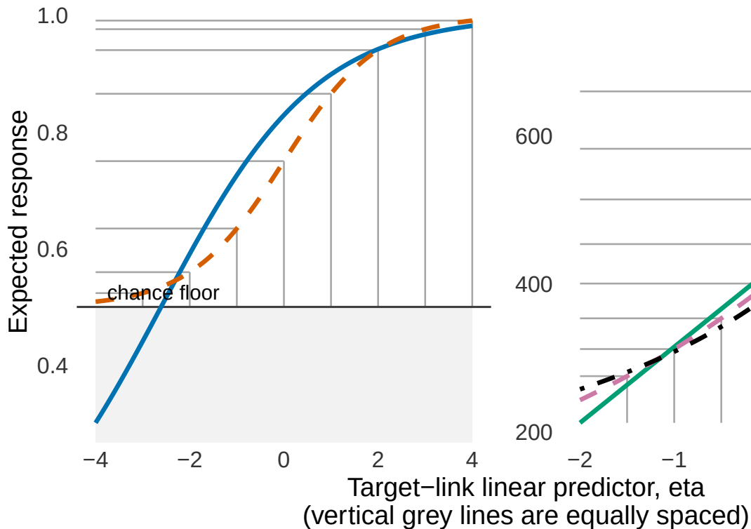
A. Binomial accuracy
