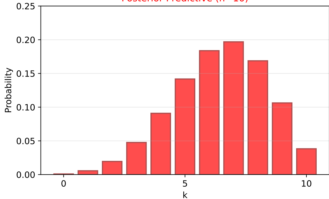
Posterior Predictive (n=10)
