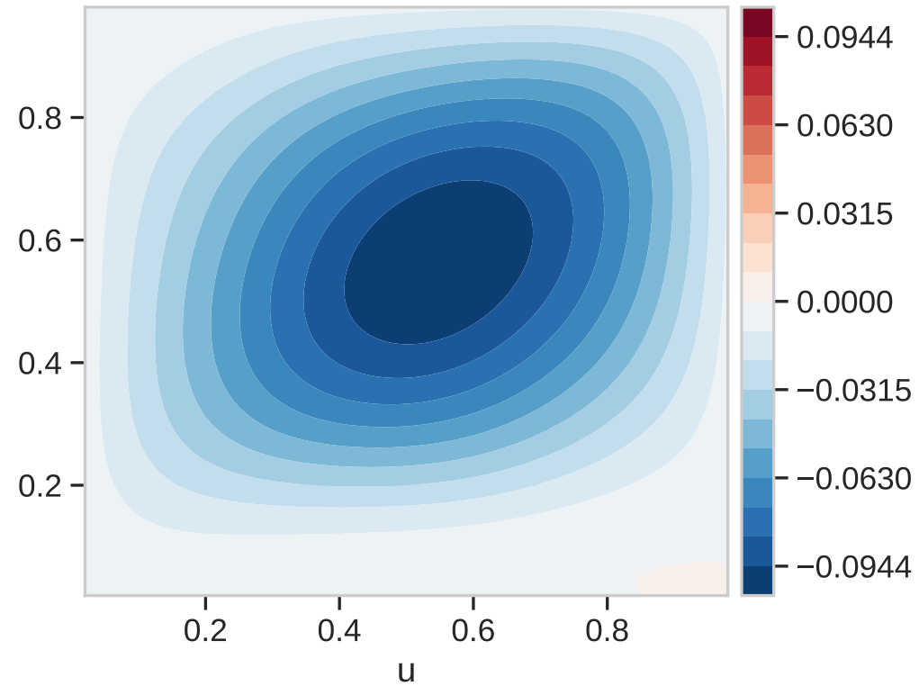
Difference (Bernstein - True)
