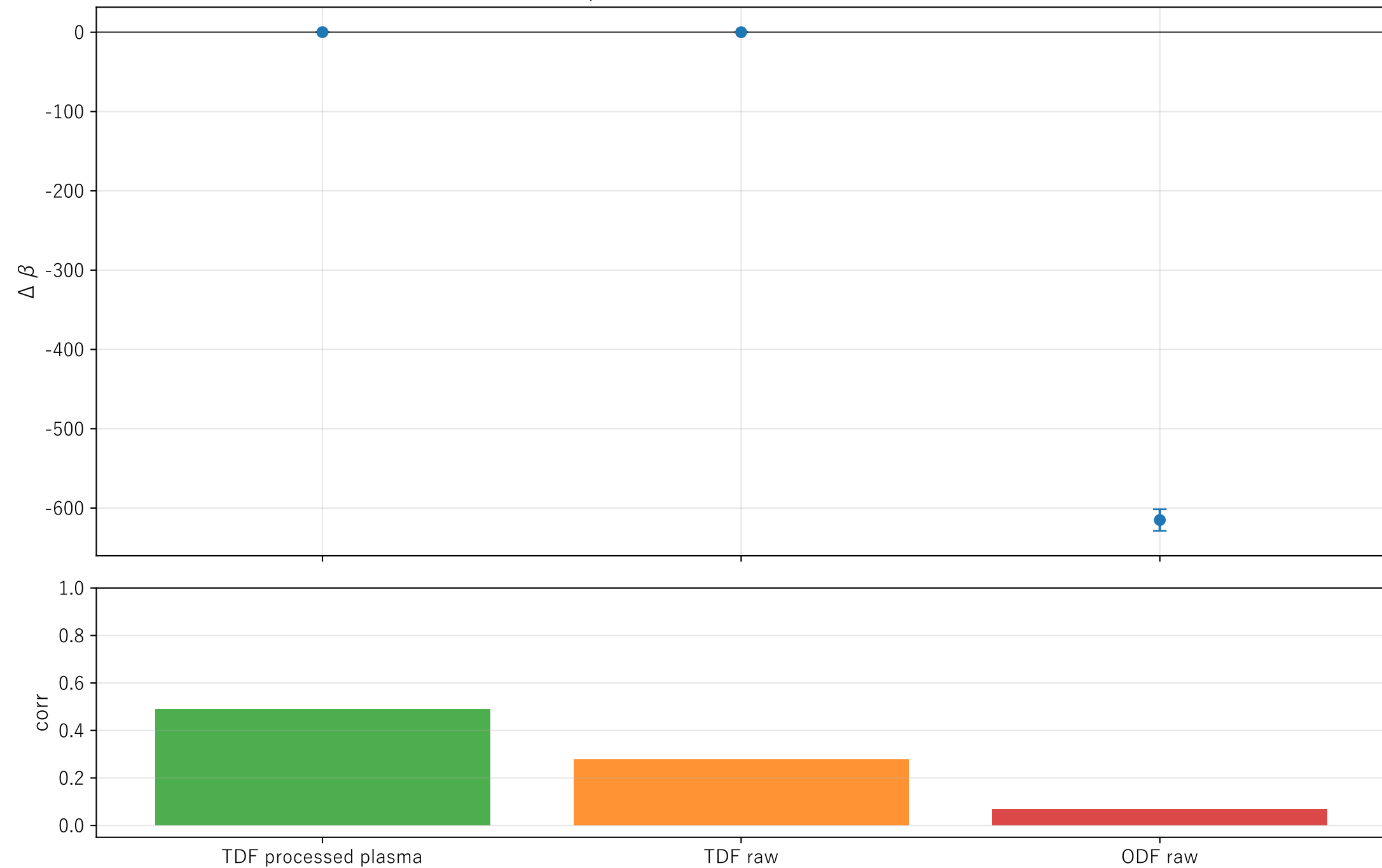
Cassini 直接 \beta fitの前処理依存比較 (同一窓・同一式)
