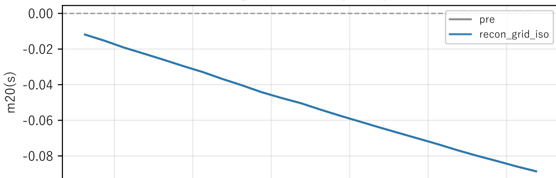
b1: 窓幅 mixing 係数 m_{20} ( \xi_0 \rightarrow \xi_2 への漏れ)
