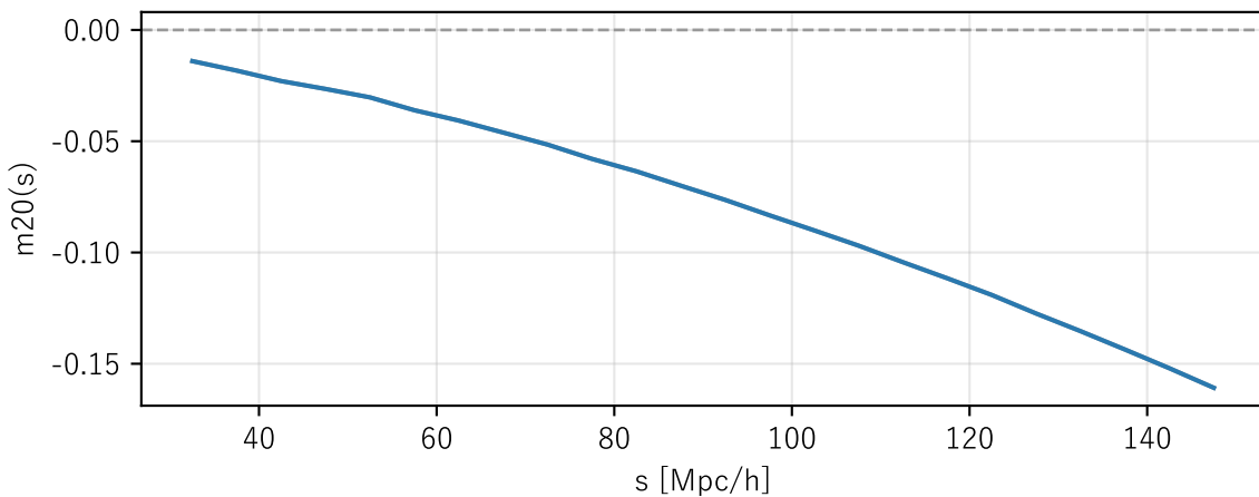
b3: 窓幅 mixing 係数 m_{20} ( \xi_0 \rightarrow \xi_2 への漏れ)
