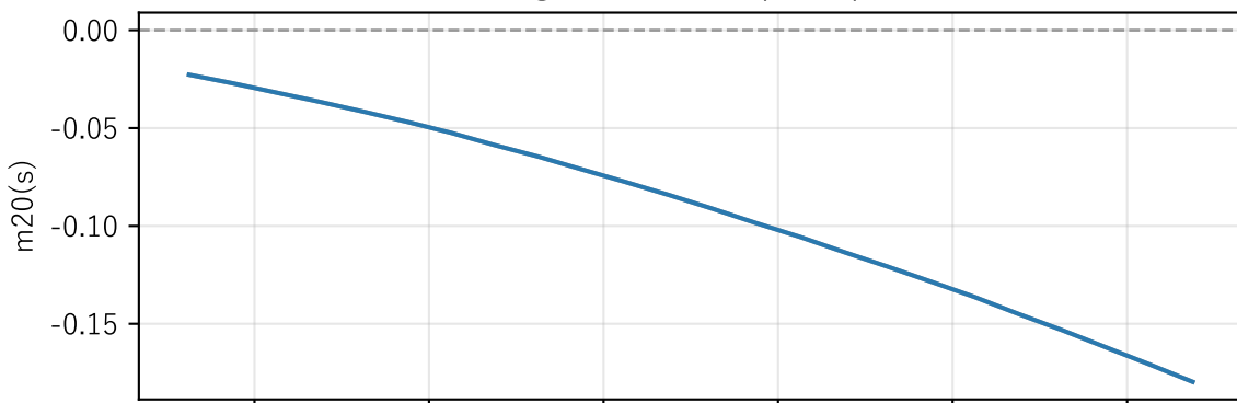
b2: 窓幅 mixing 係数 m_{20} ( \xi_0 \rightarrow \xi_2 への漏れ)
