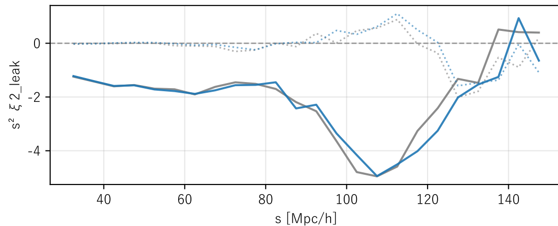
b3: 推定漏れ s^2(m_{20} \cdot \xi_0)
