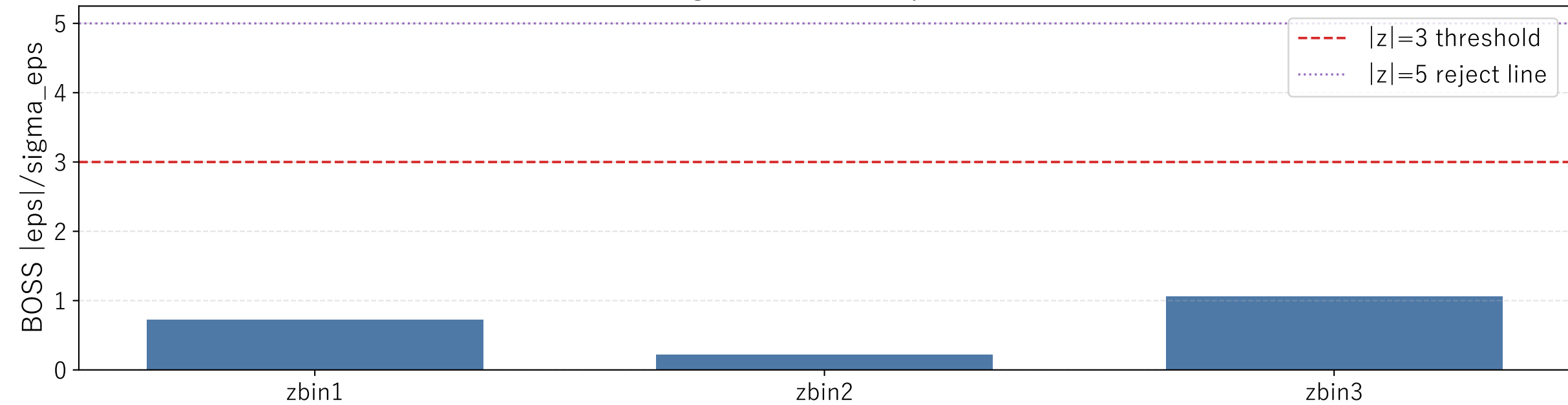
Stage A: BOSS xi_l peakfit
