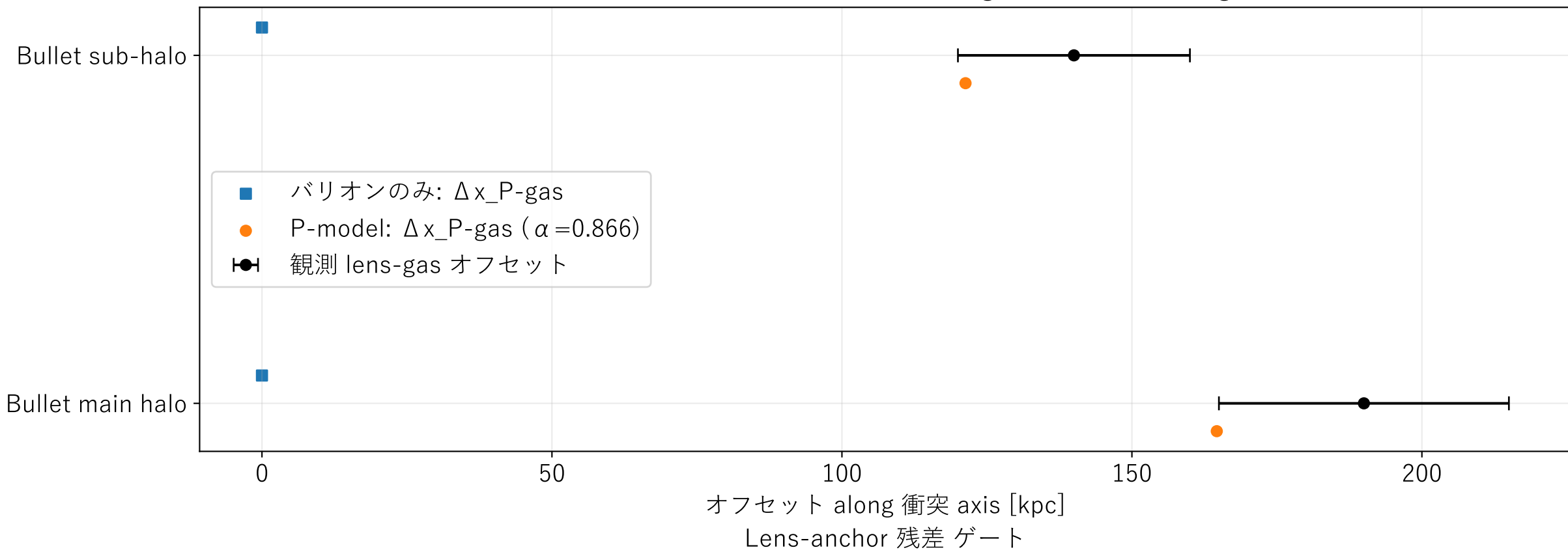
Bullet-銀河団 オフセット 監査: 観測 lens-gas 対 モデル \Delta x_{\text{P-gas}}
