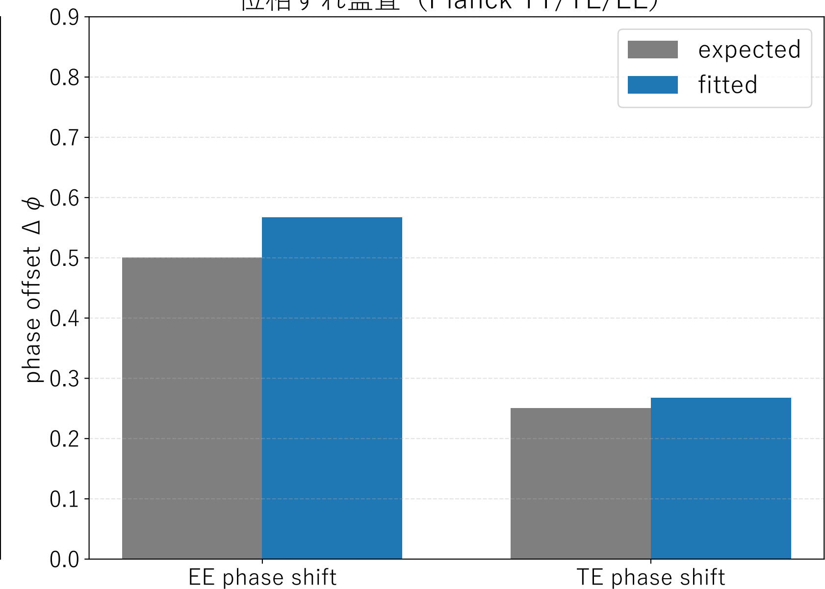
位相ずれ監査 (Planck TT/TE/EE)
