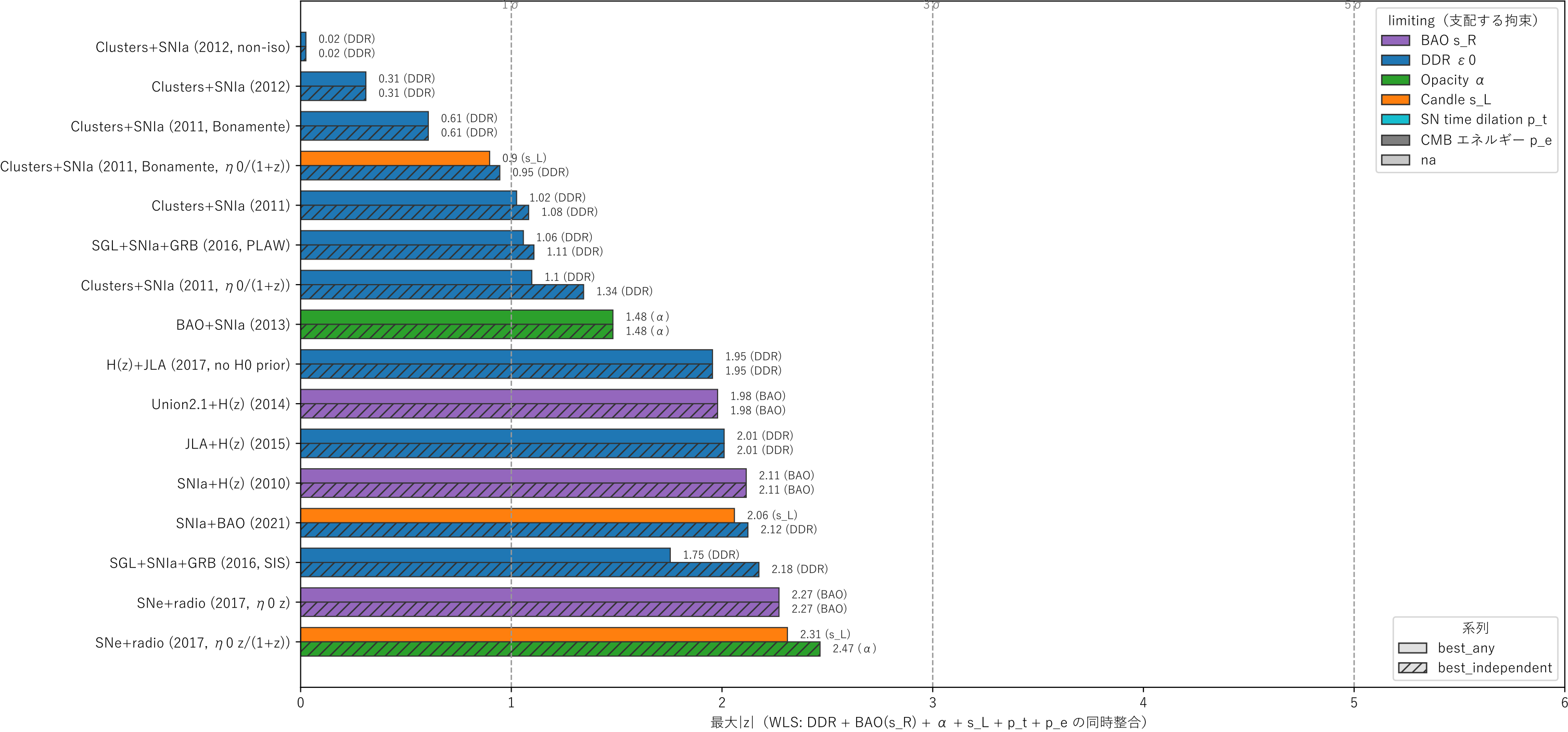
宇宙論（再接続候補探索）：支配拘束（limiting）の一覧（DDR \sigma : category_sys）
