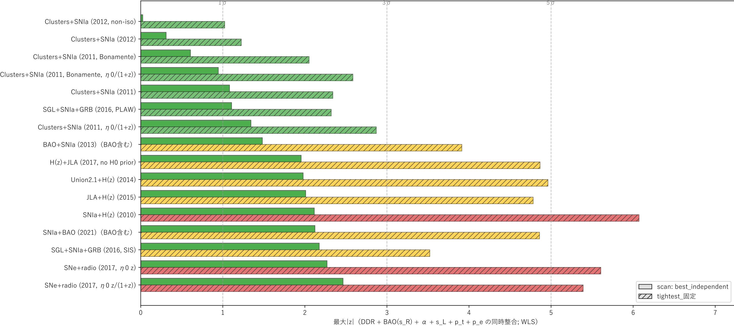
宇宙論（再接続候補探索）：一次ソース選択ルール之感度（DDR \sigma : category_sys）
