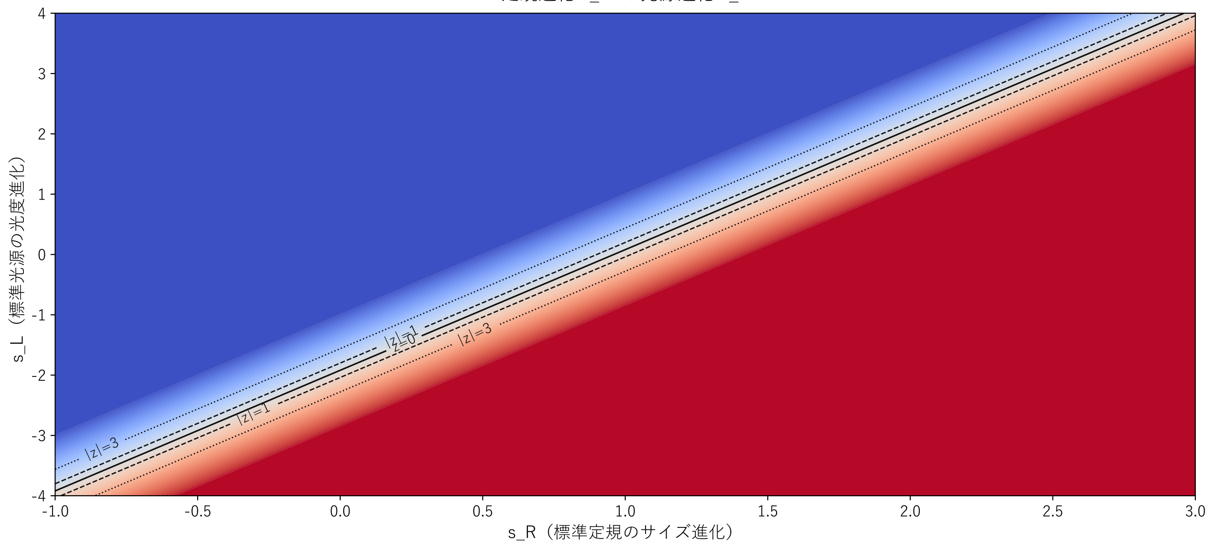
Slice C: 不透明度なし ( \alpha=0 ) 定規進化 s_R vs 光源進化 s_L
