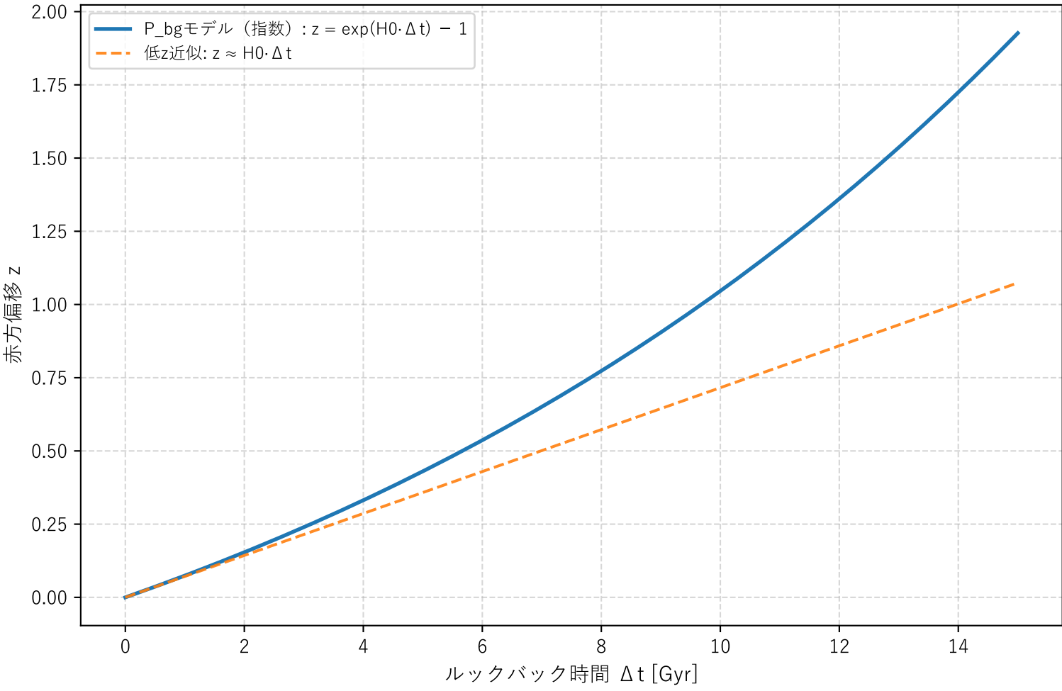
赤方偏移 z とルックバック時間 \Delta t
