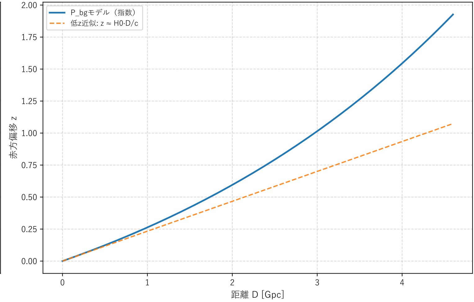
赤方偏移 z と距離 D （静的近似 D \approx c \Delta t ）
