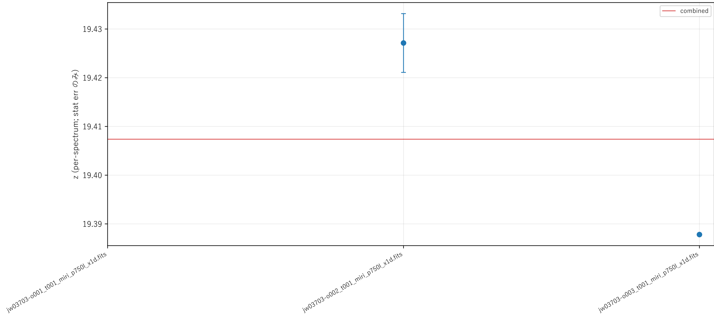
JWST z_confirmed 要約 : ceers2_5429
