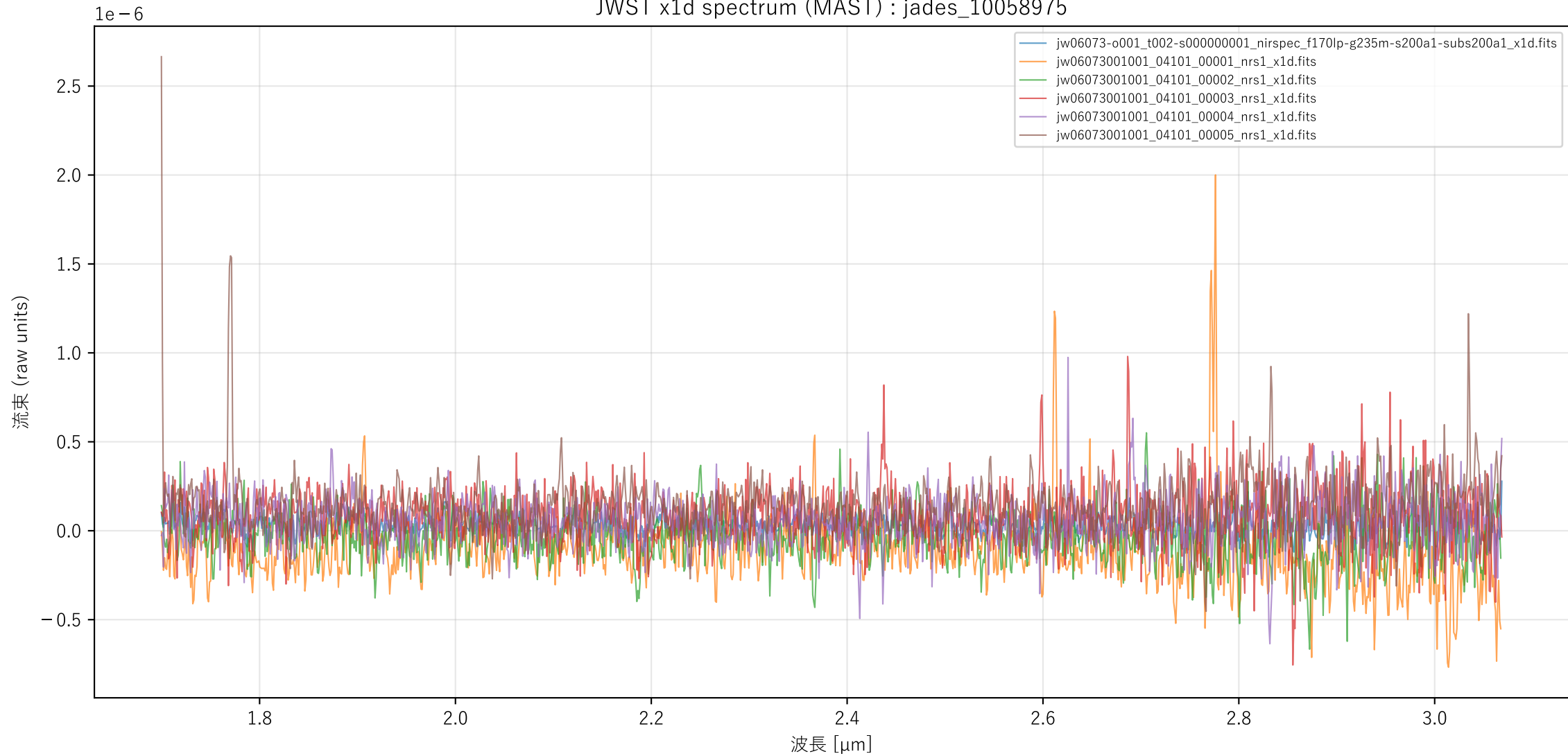
JWST x1d spectrum (MAST) : jades_10058975
