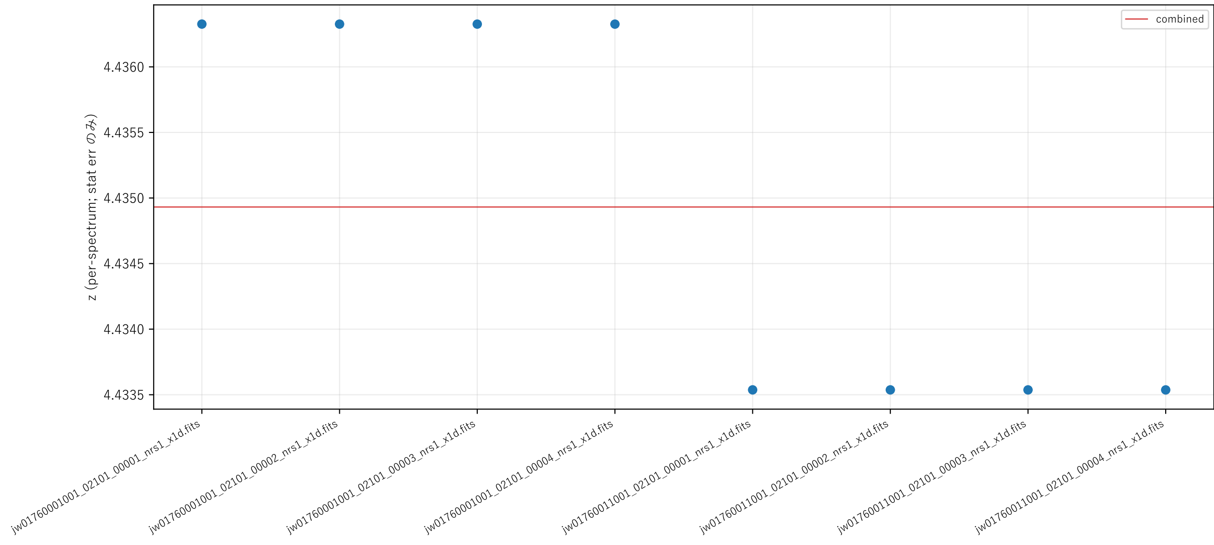
JWST z_confirmed 要約 : lid_568
