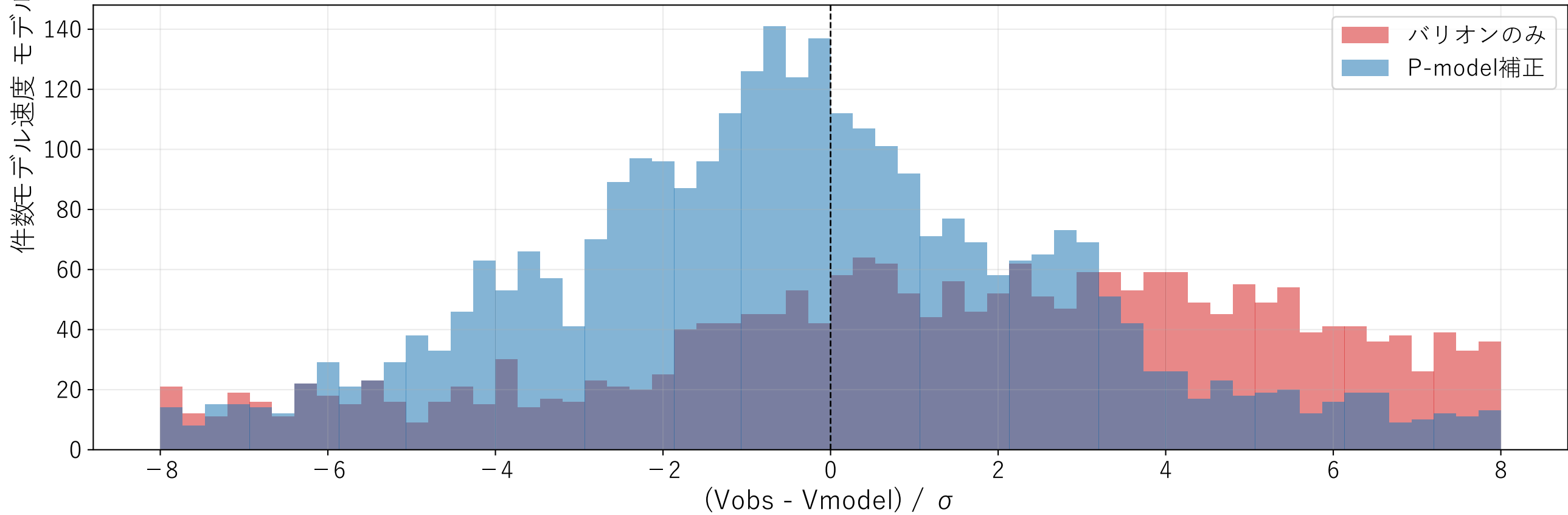
正規化残差分布
