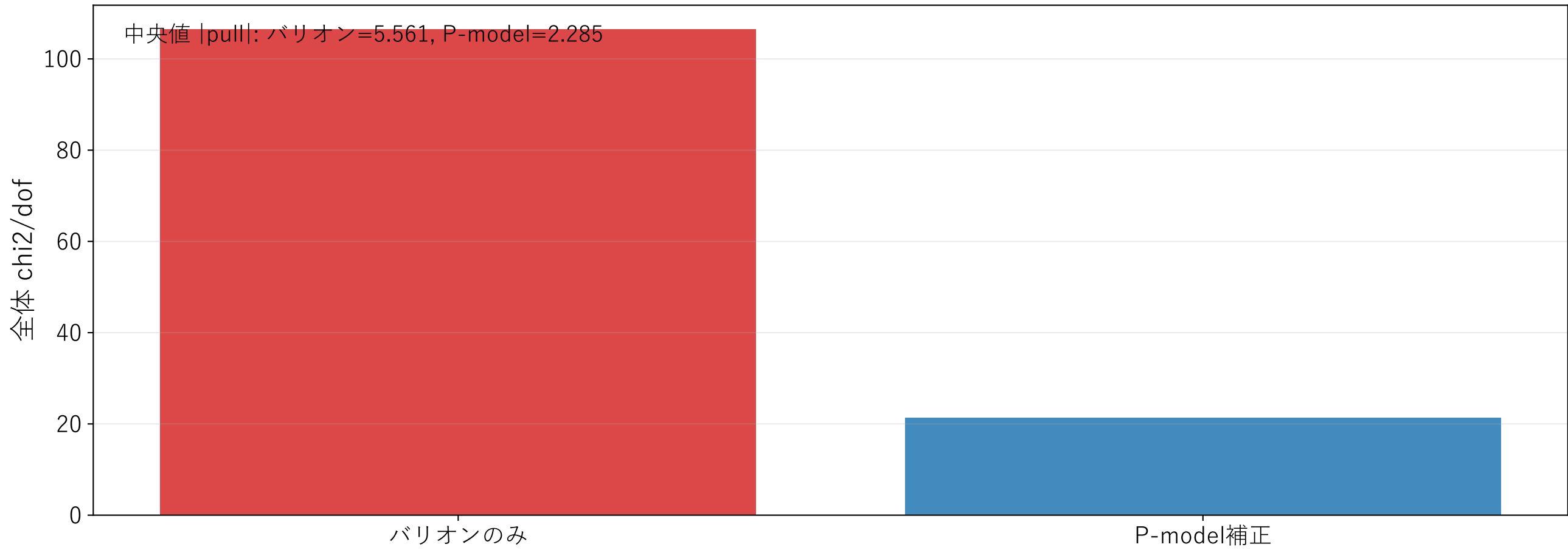
フィット品質（単一 M/L パラメータ）
