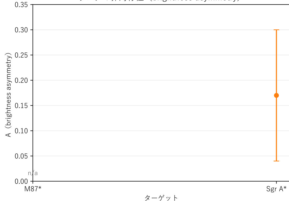
リングの非対称性（brightness asymmetry）
