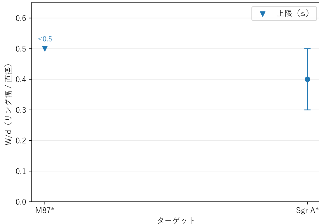
リングの幅（fractional width）
