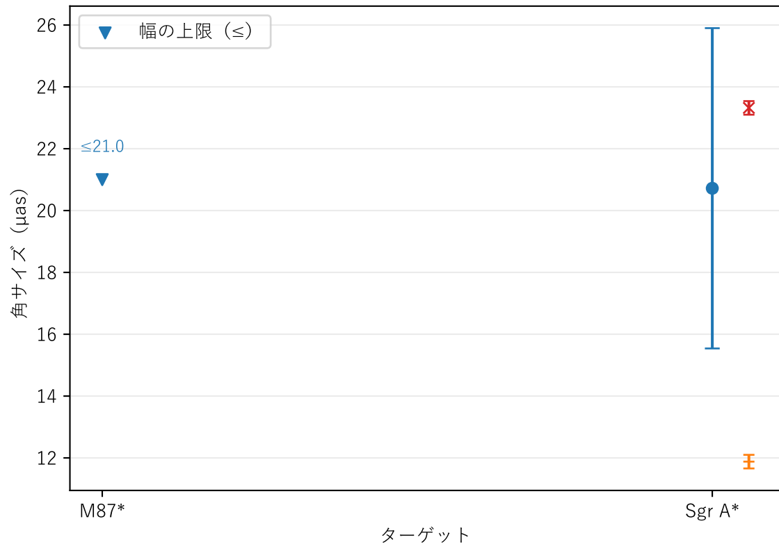
形状スケール：リング幅（ W/d \rightarrow \mu\text{as} ）と散乱blur（参考）
