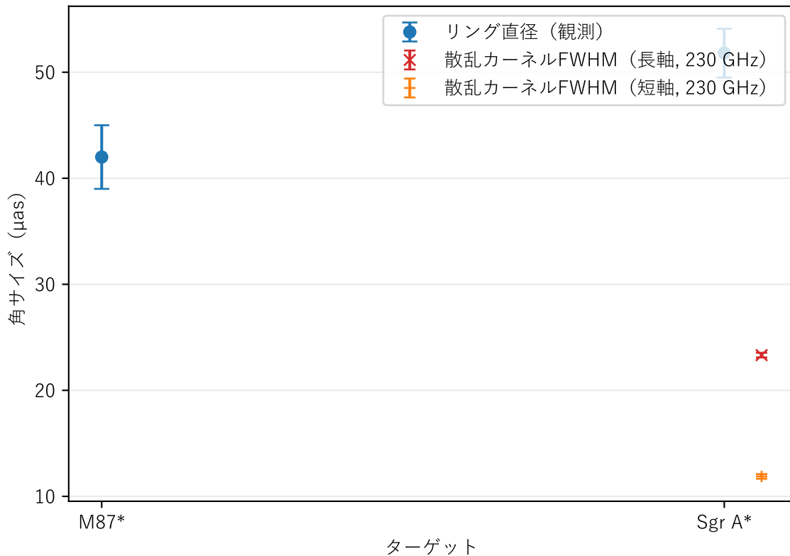
直径スケール：観測リングと散乱blur（参考）
