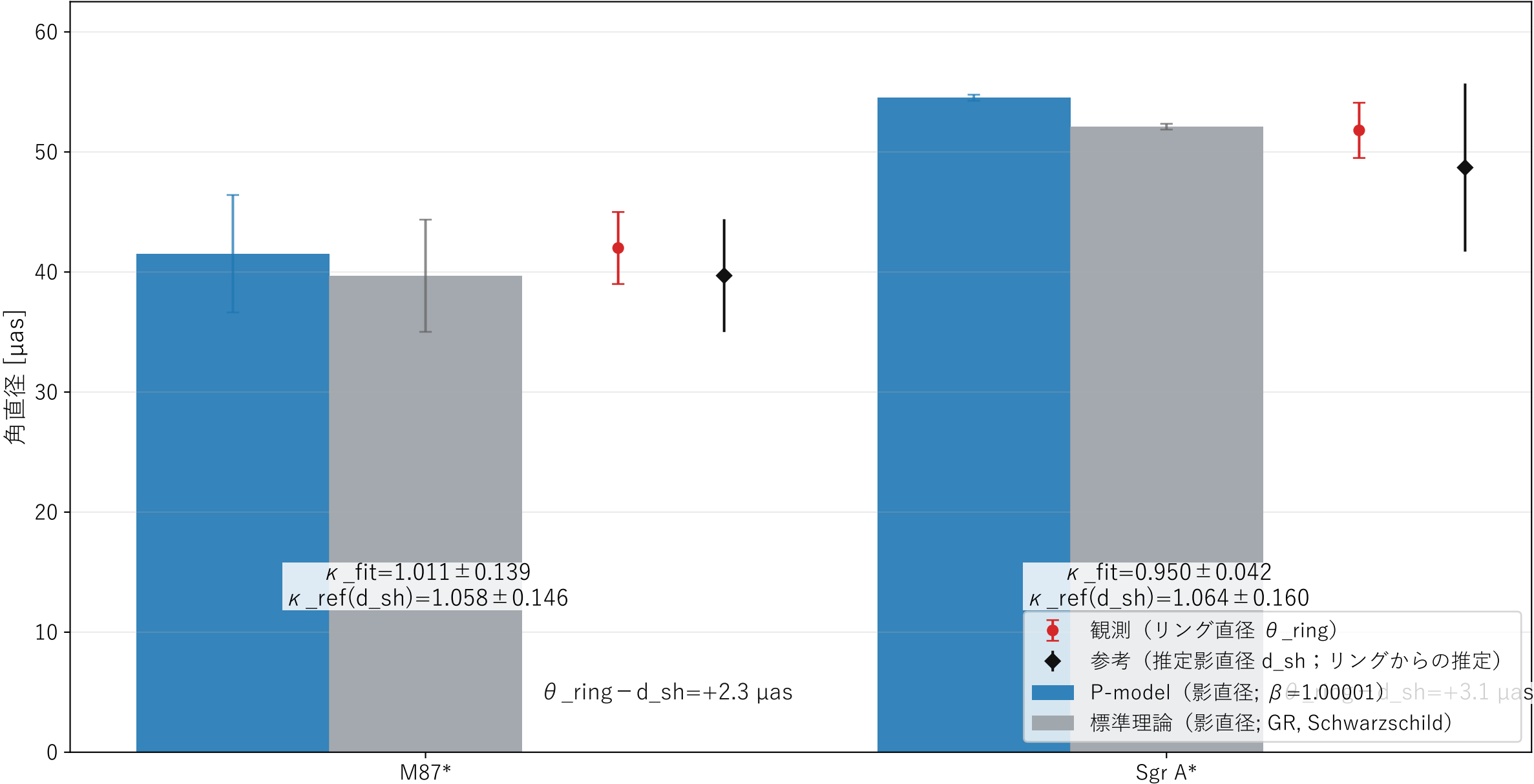
EHT：観測リング \theta_{\text{ring}} と、影直径 \theta_{\text{sh}} （モデル； \kappa=1 ）の比較
