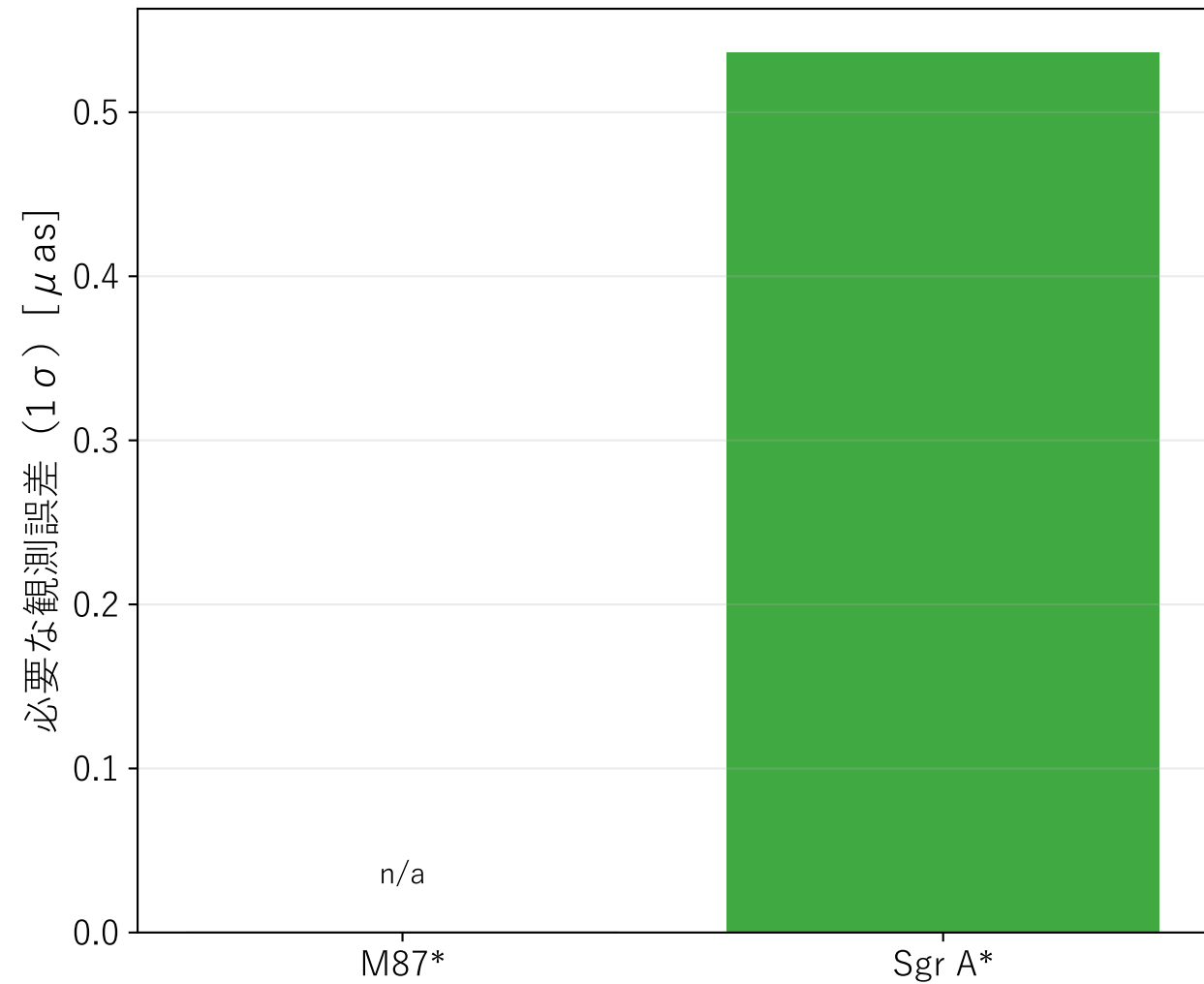
3\sigma で判別するための必要精度（目安）
