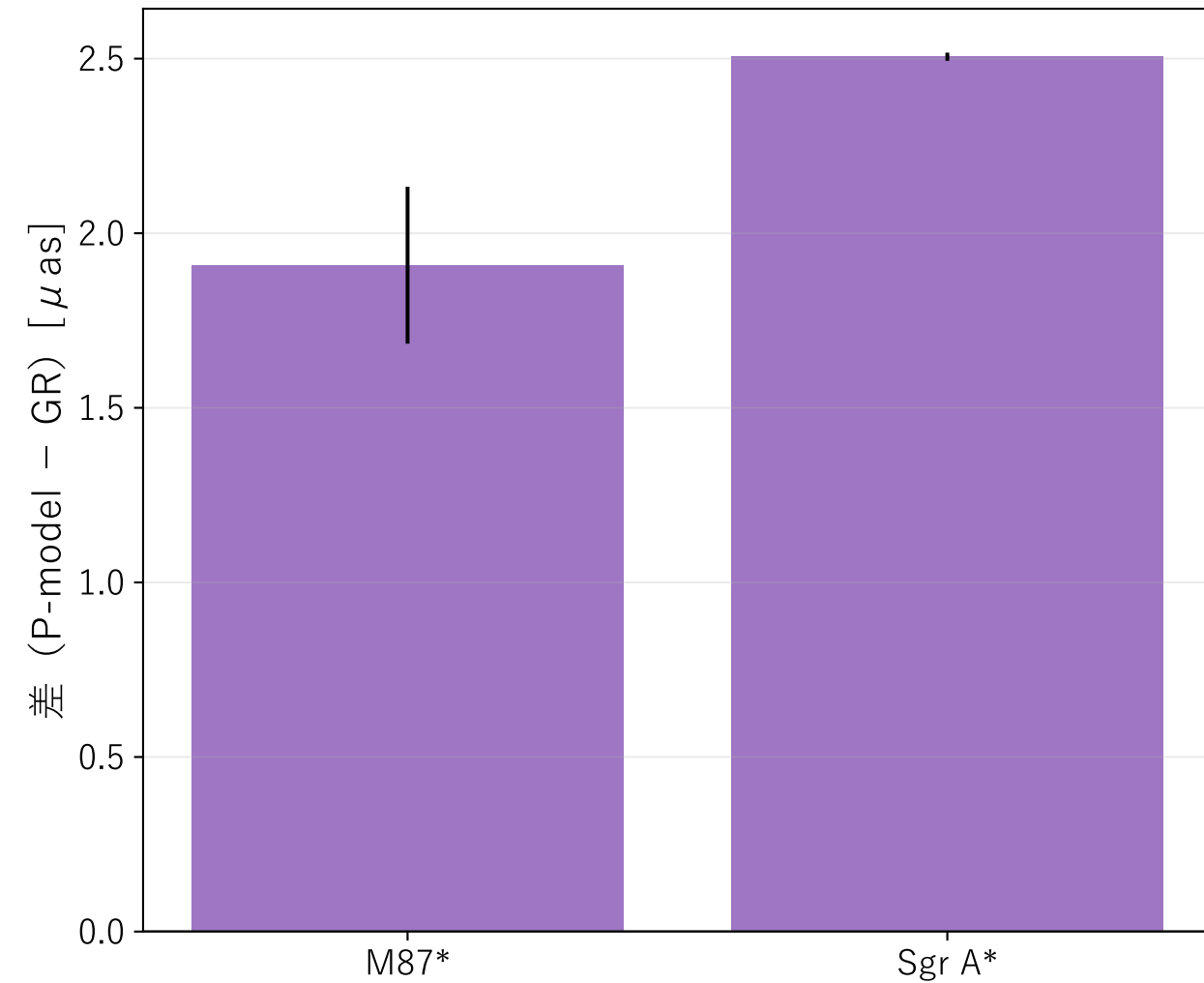
差分予測：シャドウ直径の差
