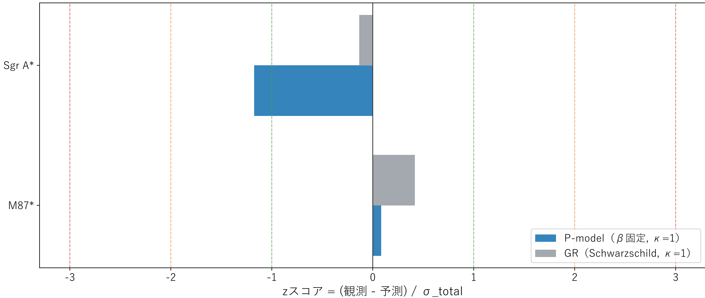
EHT：観測とモデルのずれ (zスコア, \kappa=1 の仮定)
