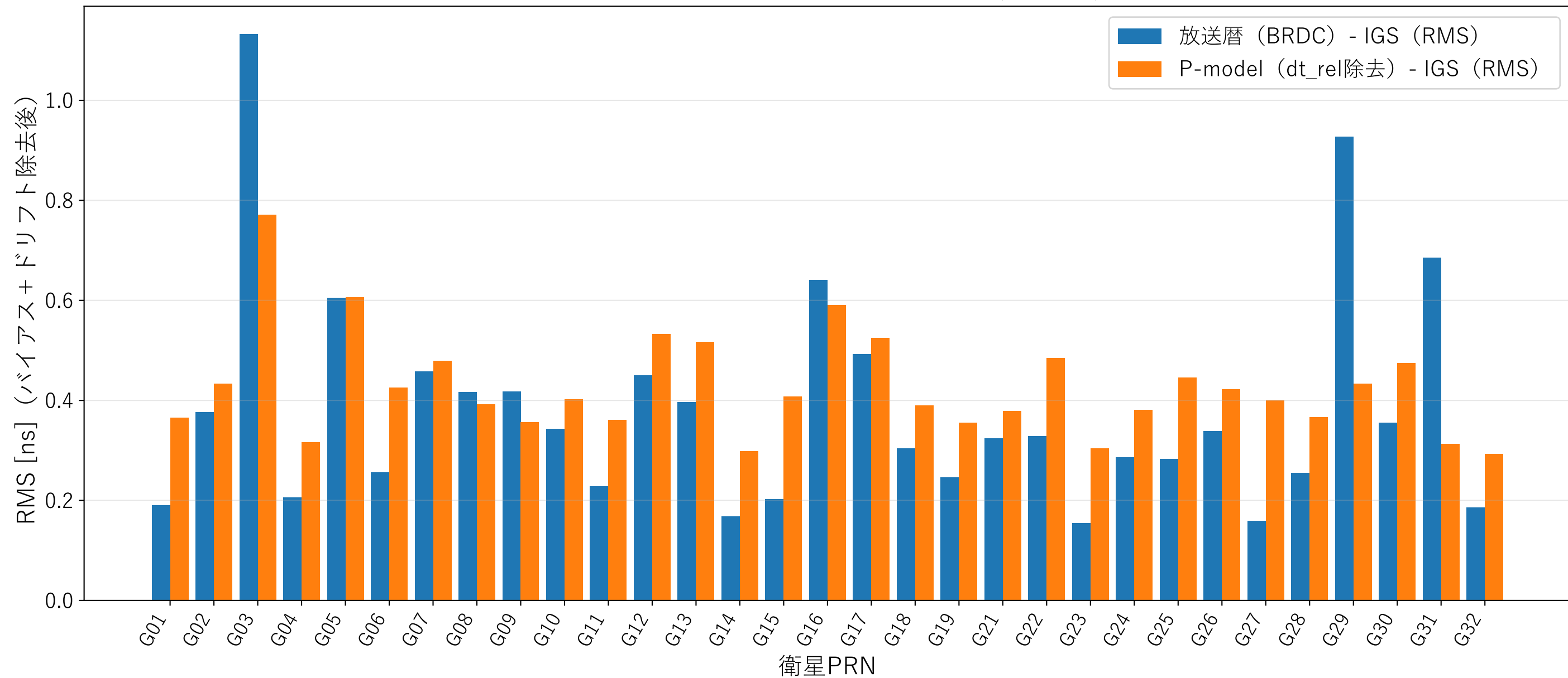
GPS：観測IGSに対する残差RMS（全衛星）
