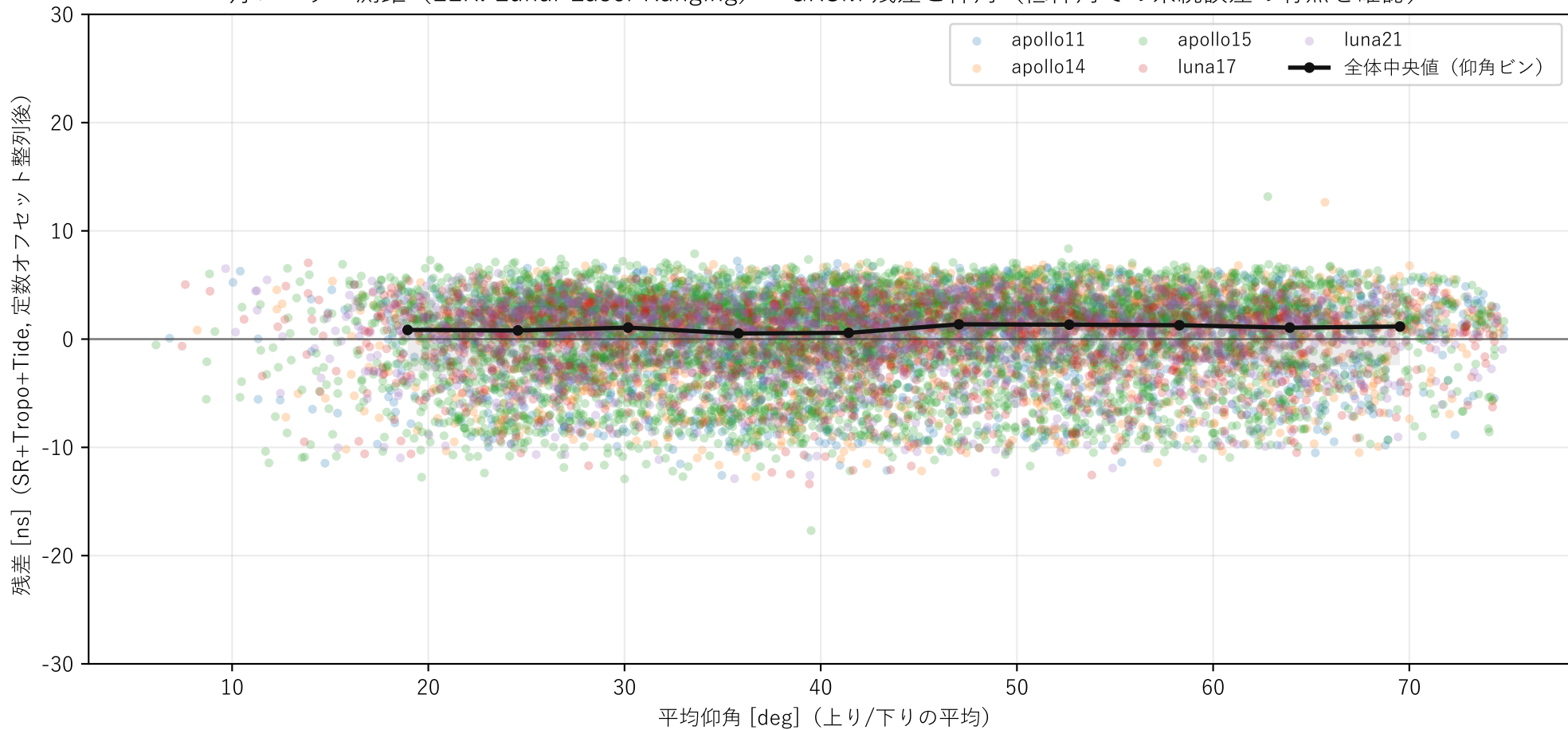
月レーザー測距（LLR: Lunar Laser Ranging）：GRSM 残差と仰角（低仰角での系統誤差の有無を確認）
