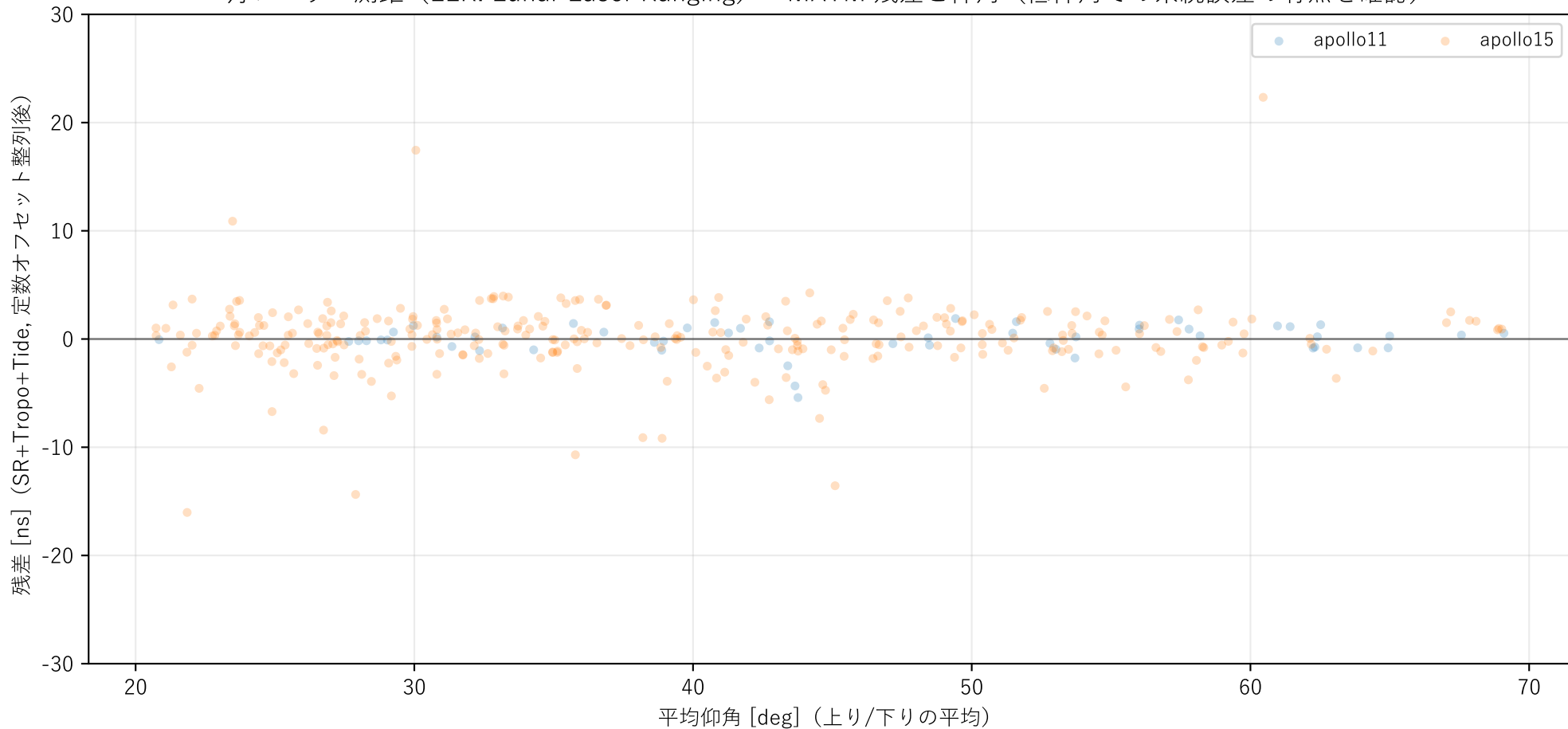
月レーザー測距（LLR: Lunar Laser Ranging）：MATM 残差と仰角（低仰角での系統誤差の有無を確認）
