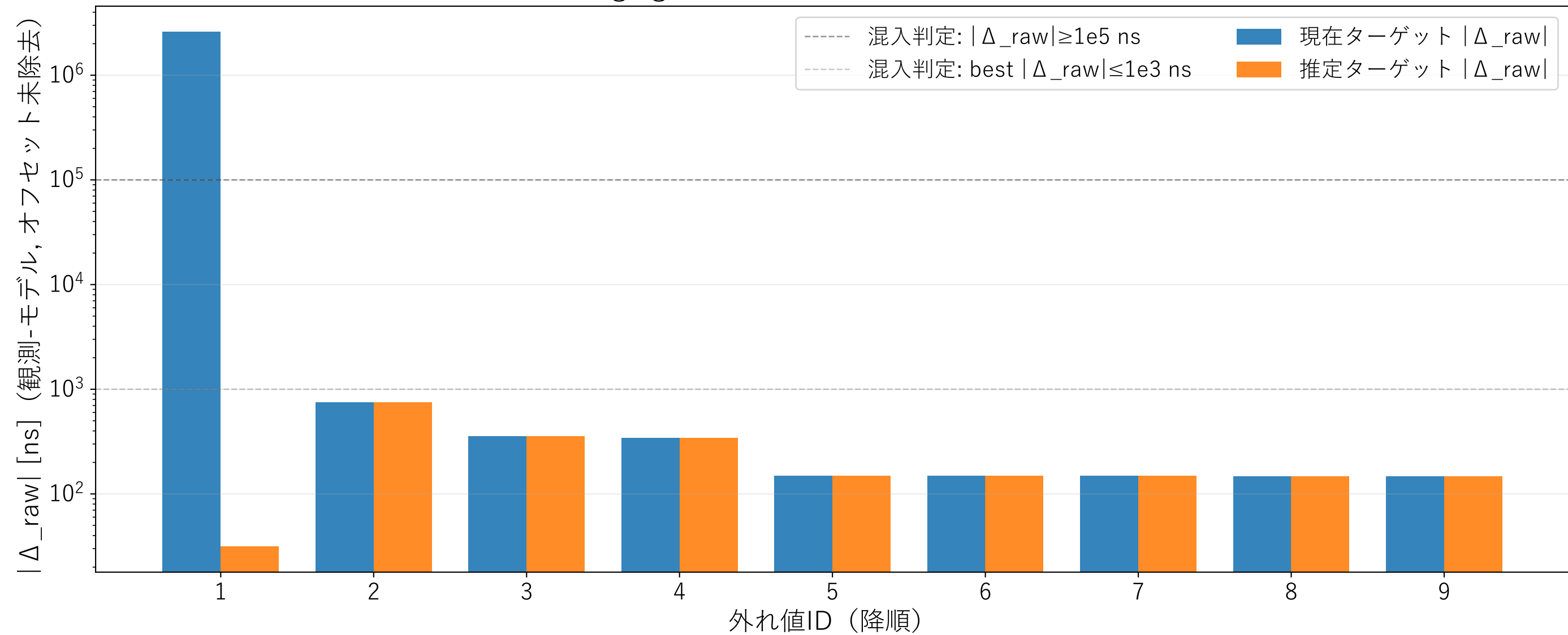
月レーザー測距（LLR: Lunar Laser Ranging）：外れ値のターゲット混入感度（現ターゲット vs 推定ターゲット）
