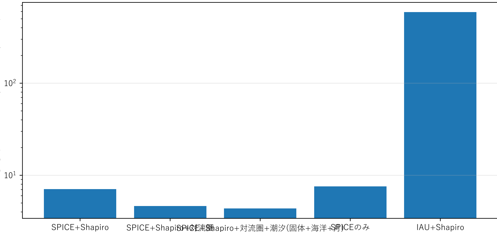
月レーザー測距（LLR: Lunar Laser Ranging）：反射器モデルの切り分け（Shapiro / 対流圏 / 潮汐 / 月回転）
