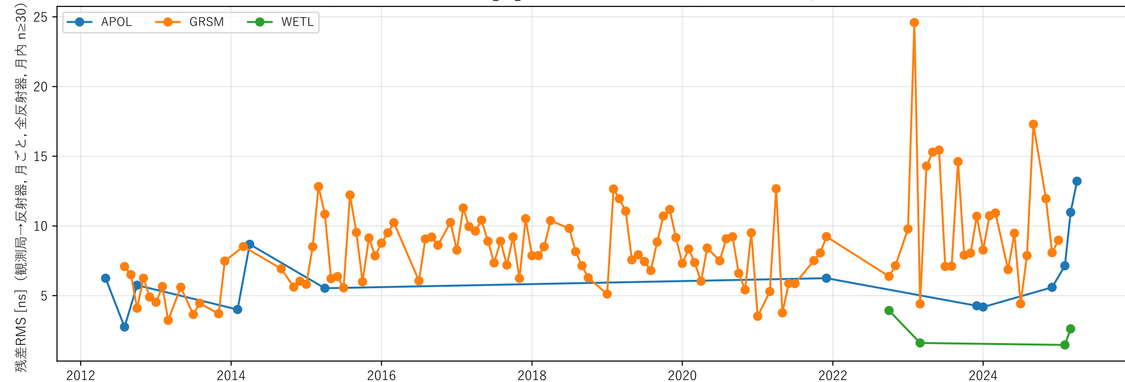
月レーザー測距（LLR: Lunar Laser Ranging）：局ごとの残差RMS（期間依存の確認, 月内 n \geq 30 のみ表示）
