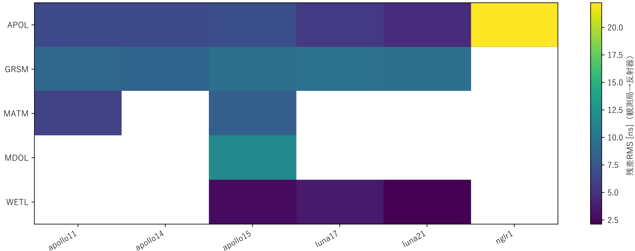
月レーザー測距（LLR: Lunar Laser Ranging）：残差RMS（観測局→反射器, 定数整列） 局 × reflector
