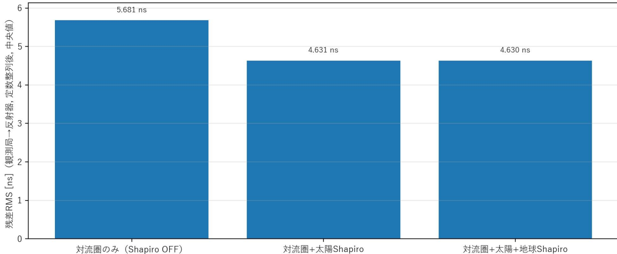
月レーザー測距（LLR: Lunar Laser Ranging）：重力遅延の寄与（ShapiroのON/OFF, 対流圏あり）
