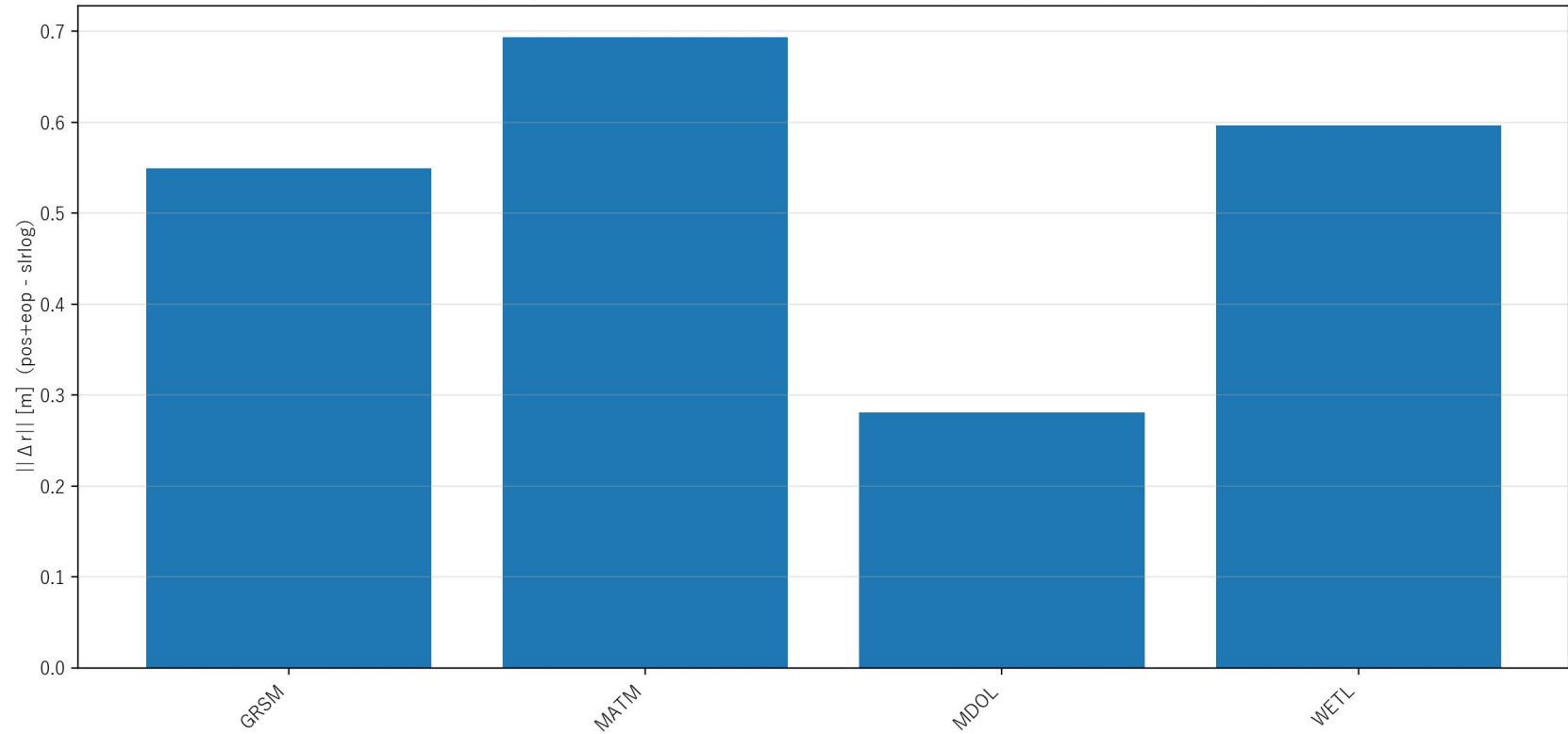
月レーザー測距（LLR: Lunar Laser Ranging）：局座標の差分（一次ソースpos+eopの影響）
