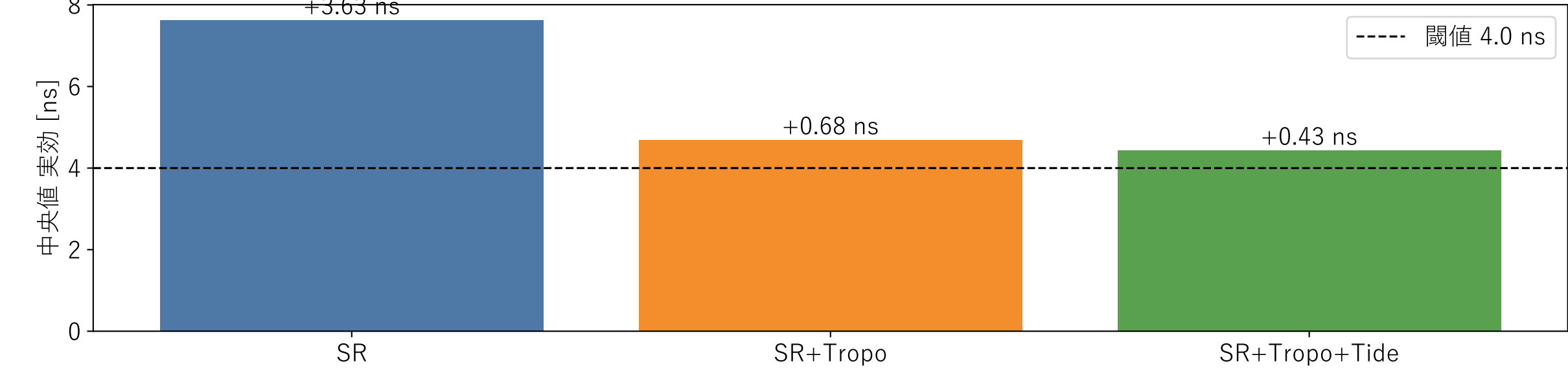
除去検証 対 4 ns 閾値
