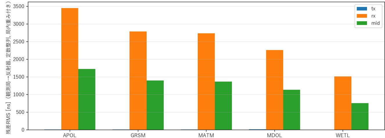
月レーザー測距 (LLR: Lunar Laser Ranging) : time-tag 最適化 (局ごとに tx/rx/mid を選択)
