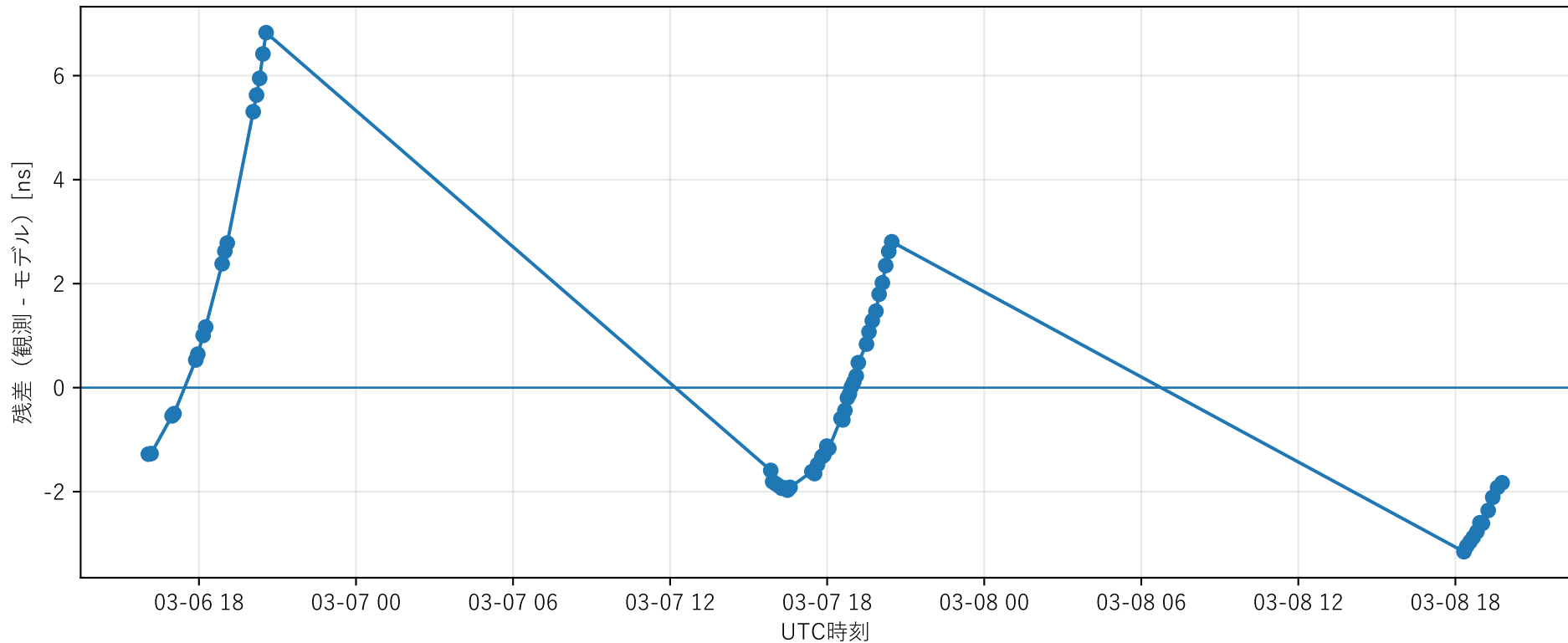
定数オフセット整列後の残差（反射器モデル, 太陽Shapiro含む）
