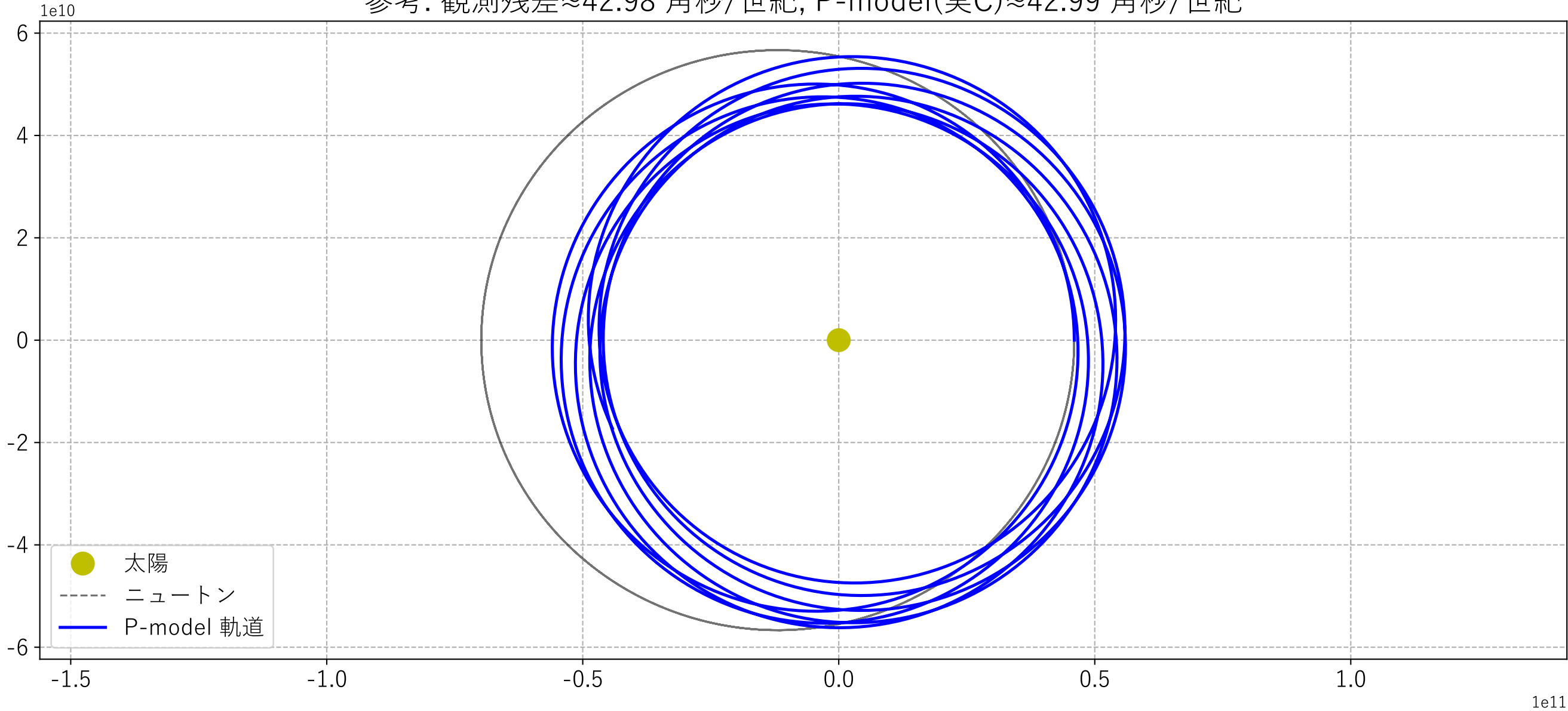
近日点移動の累積（周回ごと） （実Cでの定量評価）
