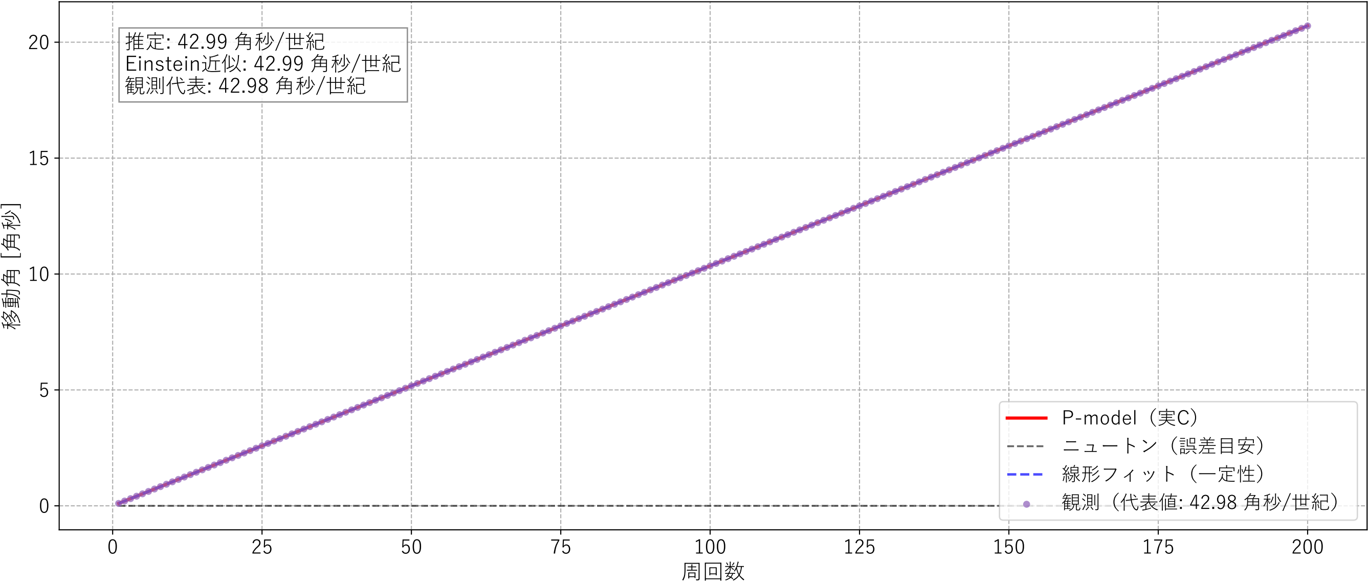
近日点移動の累積（周回ごと） （実Cでの定量評価）
