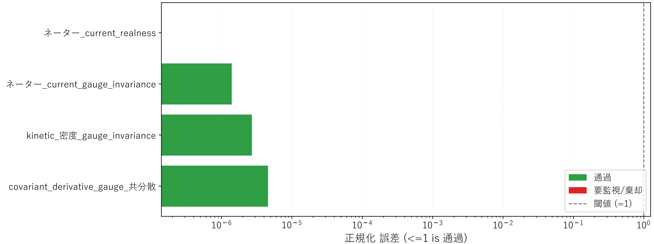
作用原理 EL 導出監査 (gauge 共分散 / invariance)
