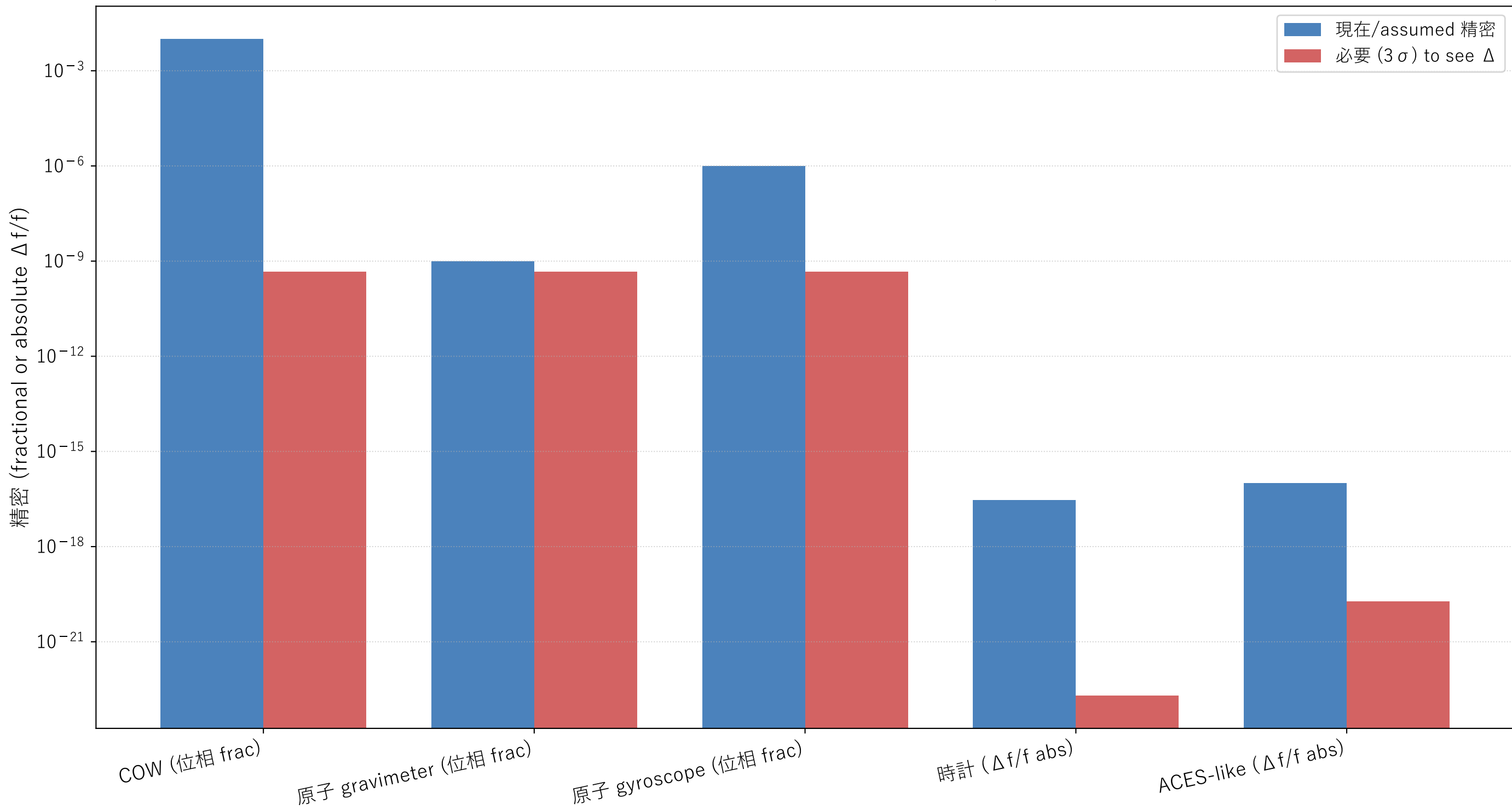
原子-interferometer 統合 監査 (P-model 対 GR; Earth field)
