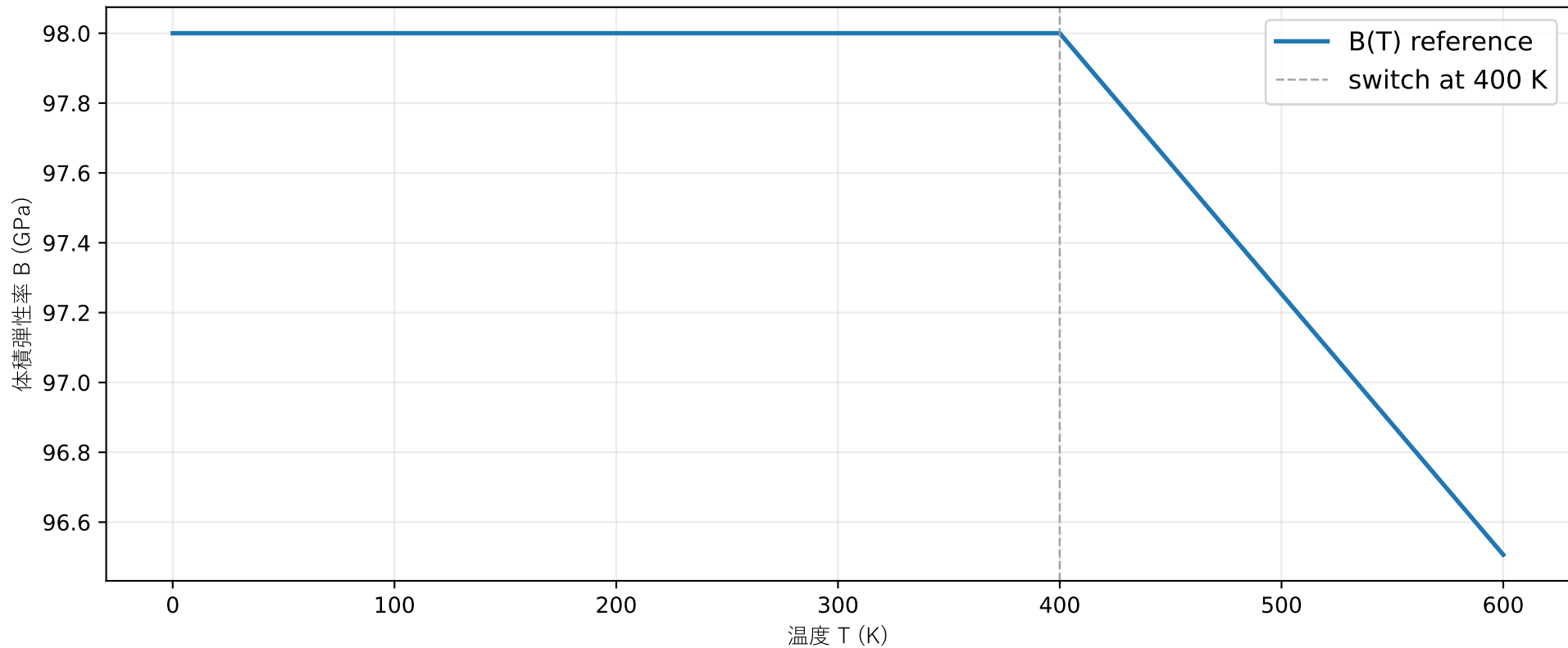
シリコン 体積弾性率 B(T) (loffe elastic constants reference)
