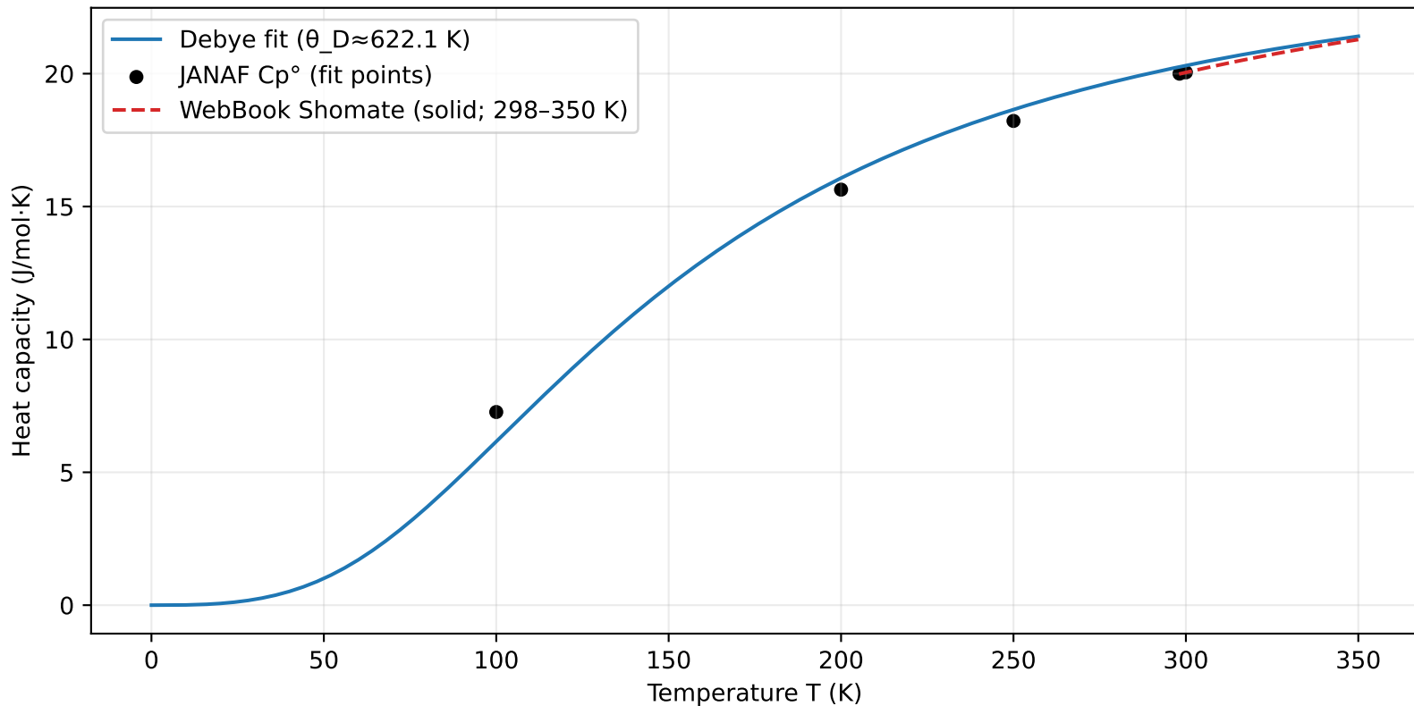
シリコン 熱容量: JANAF 基準 + Debye-fit 目標 (low T)
