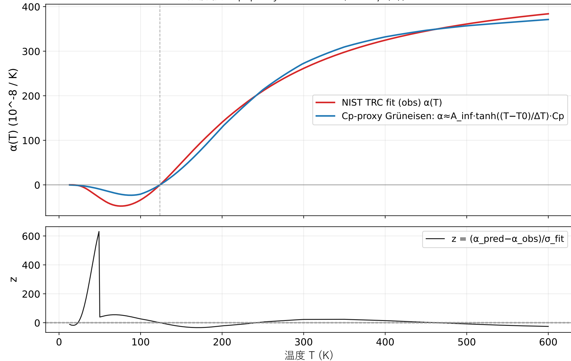
シリコン 熱膨張: Cp-proxy Grüneisen ( \tanh \gamma(T) ) ansatz check
