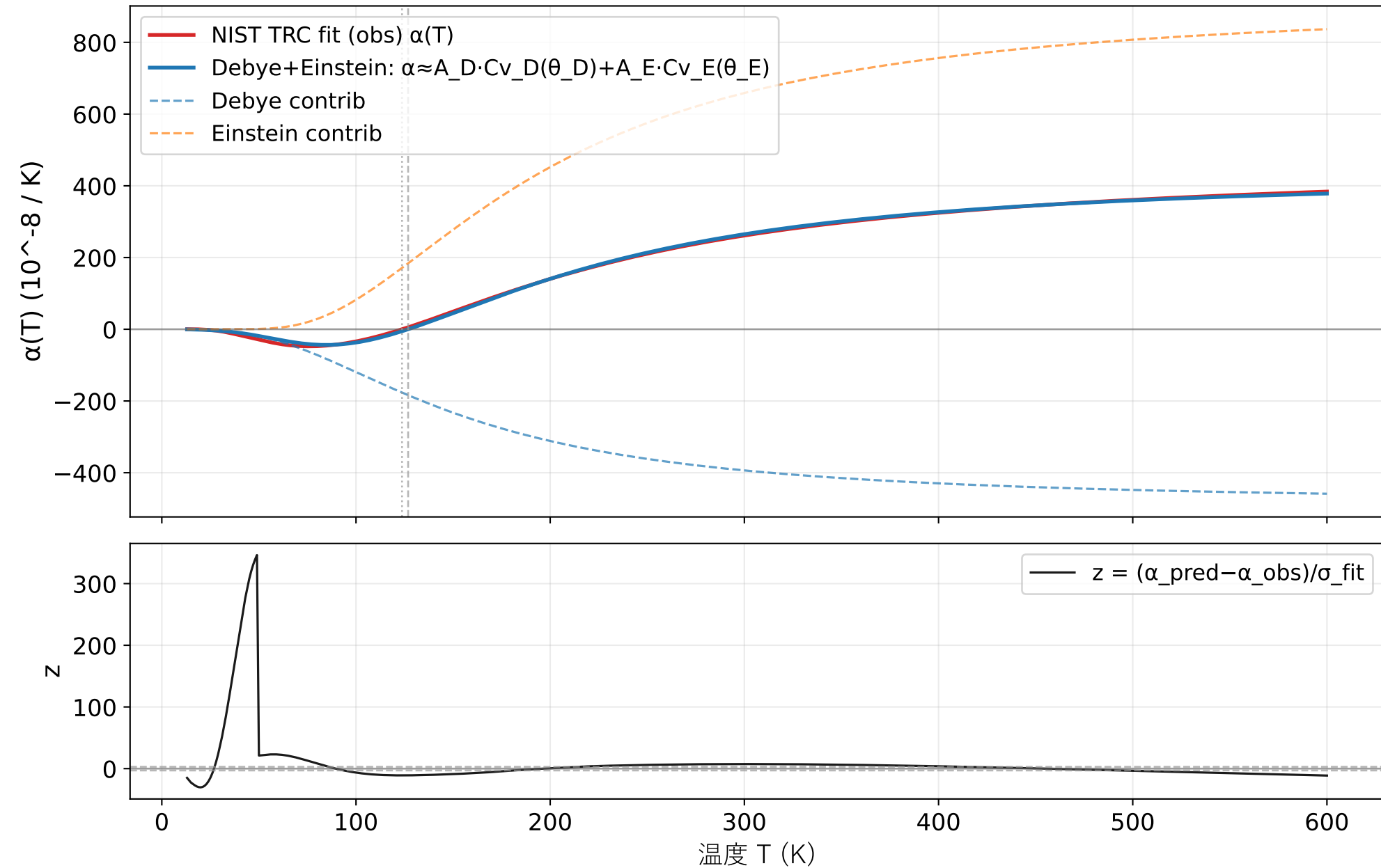
シリコン 熱膨張: Debye+Einstein (optical) ansatz check
