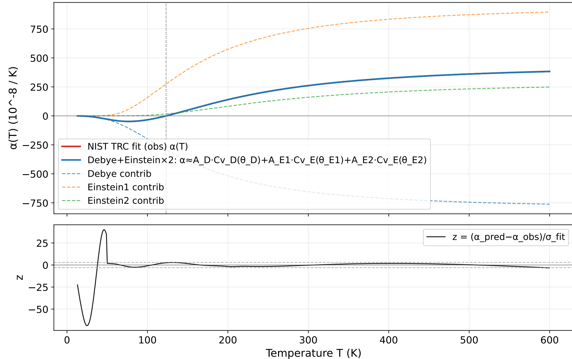
シリコン 熱膨張: Debye+Einstein×2 (two optical branches) ansatz check
