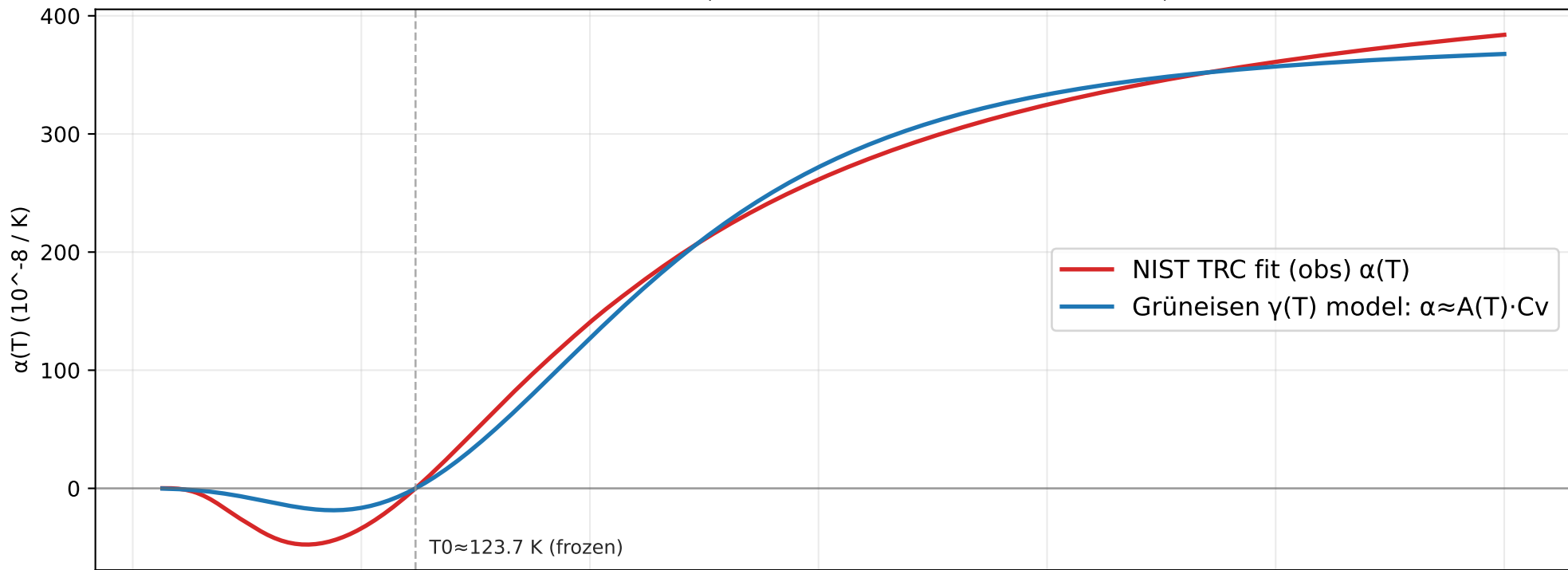
シリコン 熱膨張: minimal \gamma(T) (Grüneisen) extension (tanh interpolation)
