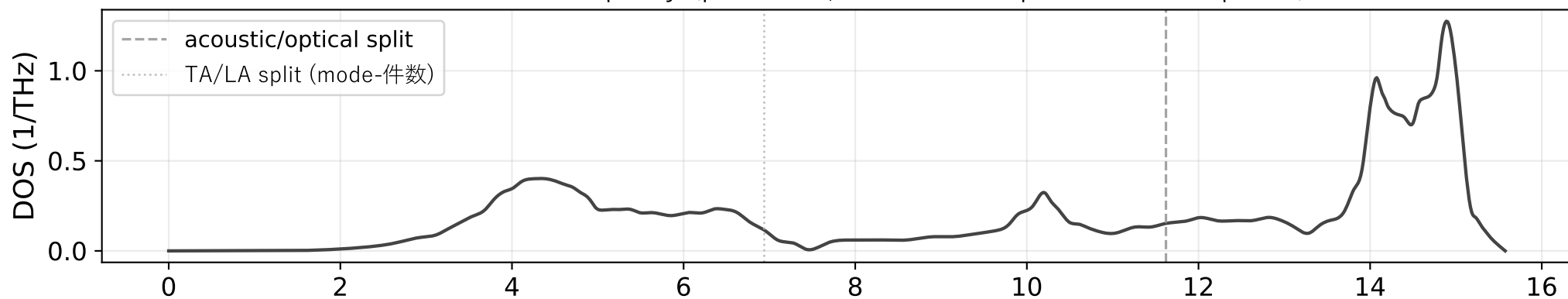
Si 熱膨張: フォノン DOS constrained Gruneisen check
