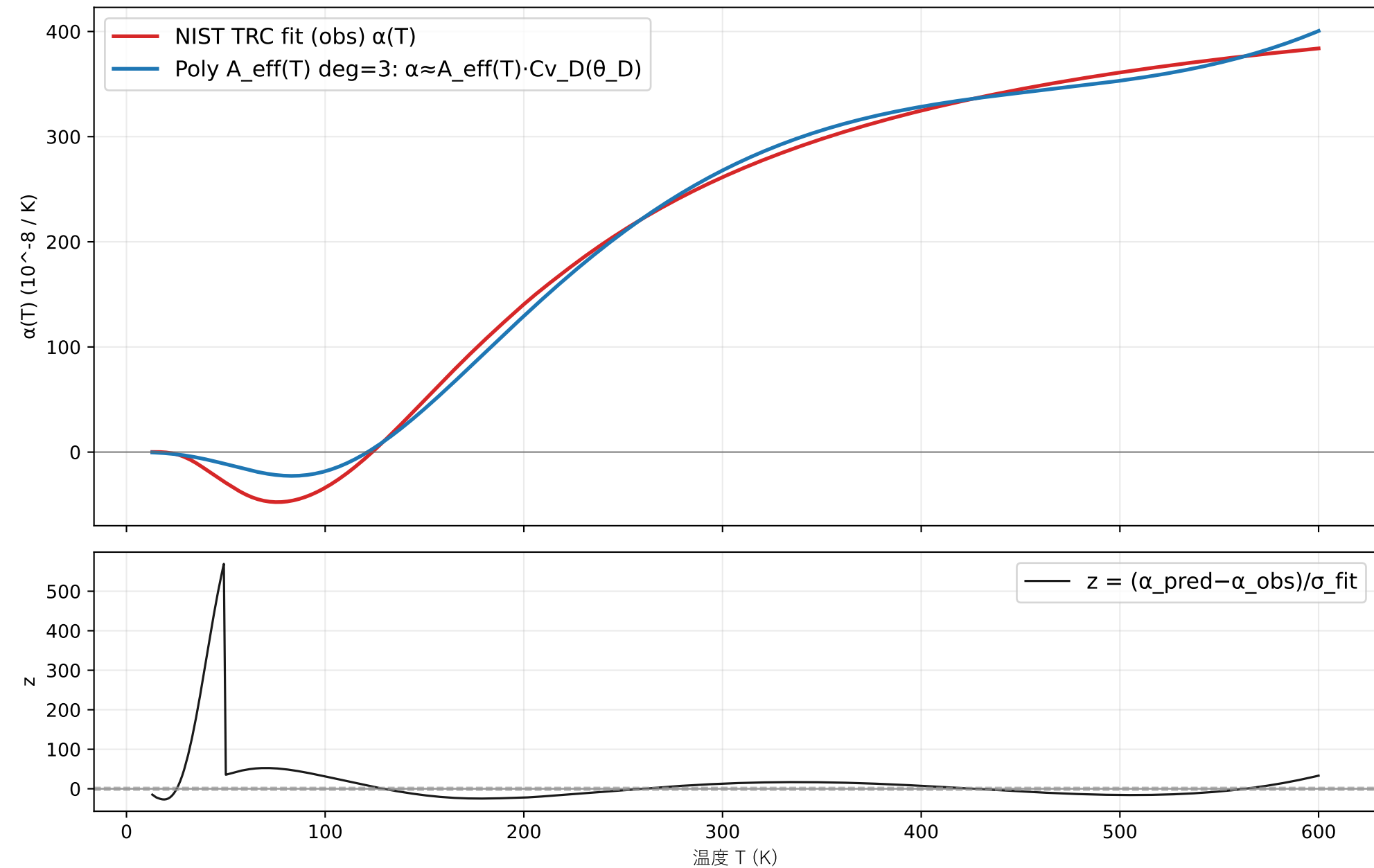
シリコン 熱膨張: polynomial A_eff(T) ansatz (diagnostic)
