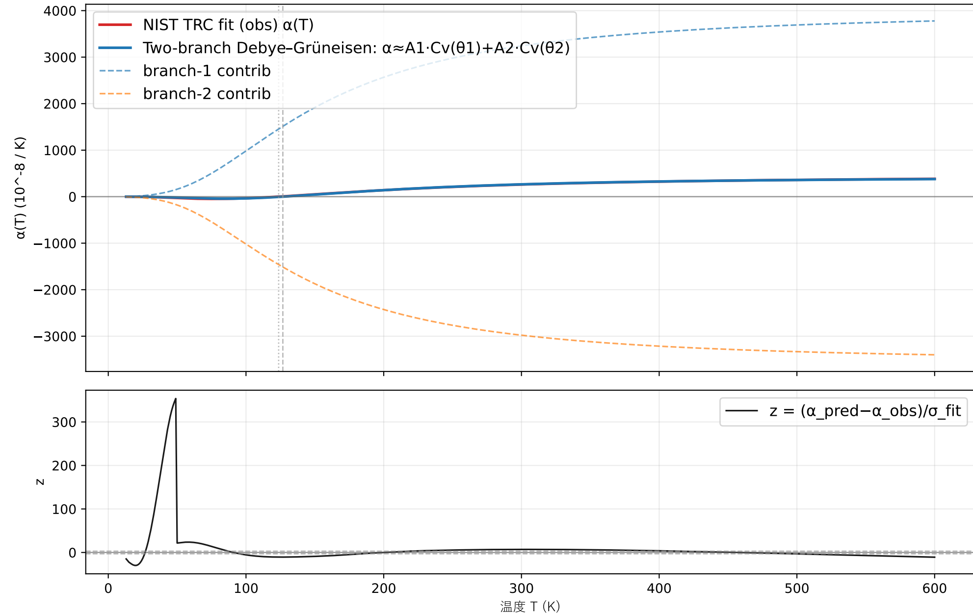
シリコン 熱膨張: two-branch Debye-Grüneisen ansatz check
