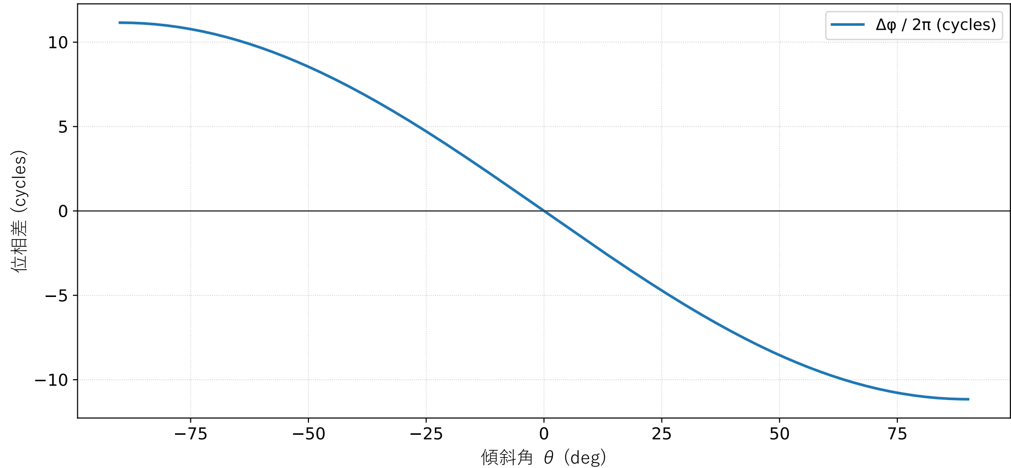
COW (重力誘起 quantum 干渉): 位相差 スケーリング
